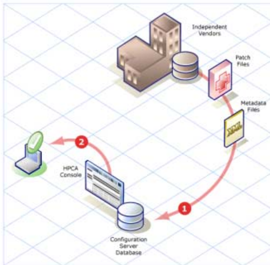
Figure 2 Modèle de gestion des correctifs - classique
