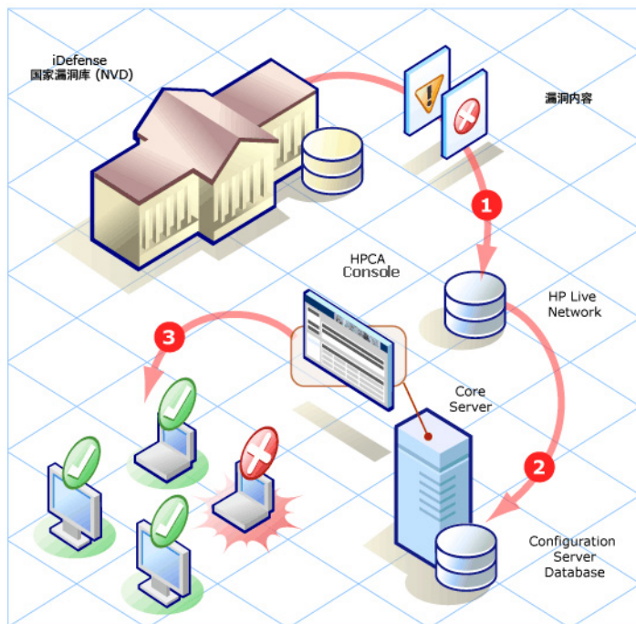
图 4 示例：HPCA 的漏洞管理
