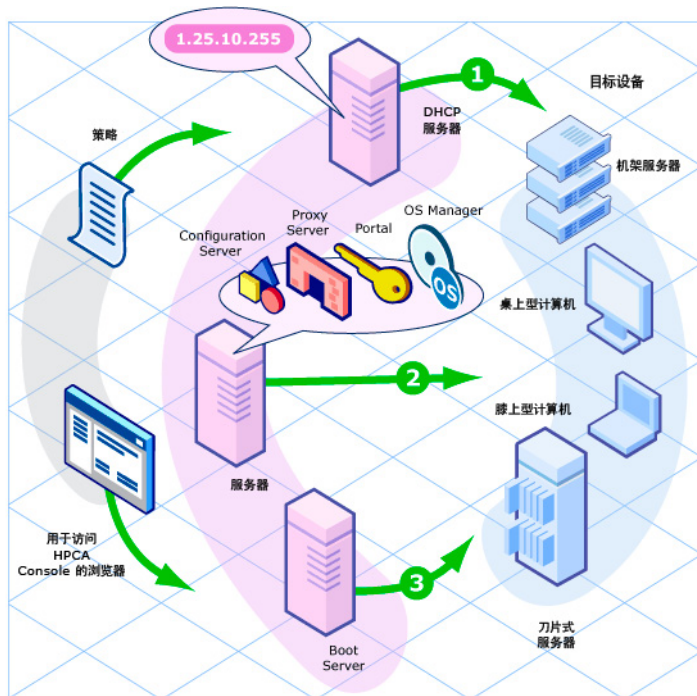
图 5 HPCA 中的 OS Manager 部署体系结构
