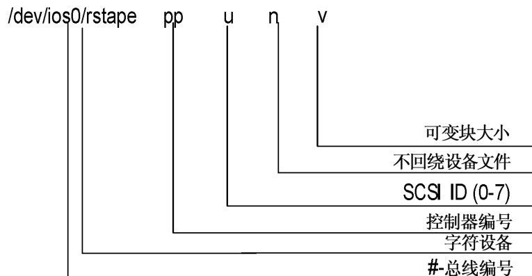
图 22 设备文件名的格式:
