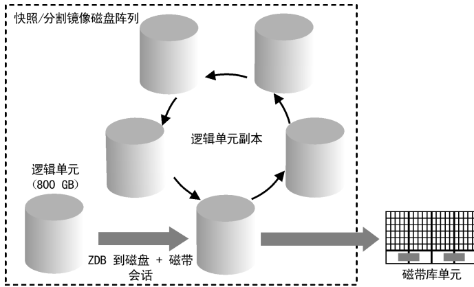
图 52 ZDB 到磁盘 + 磁带会话
