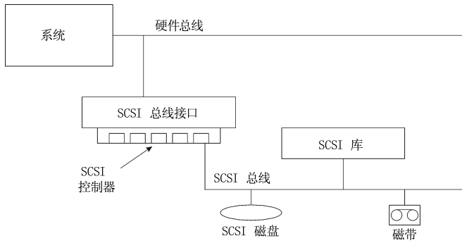
图 75 SCSI 控制的设备
