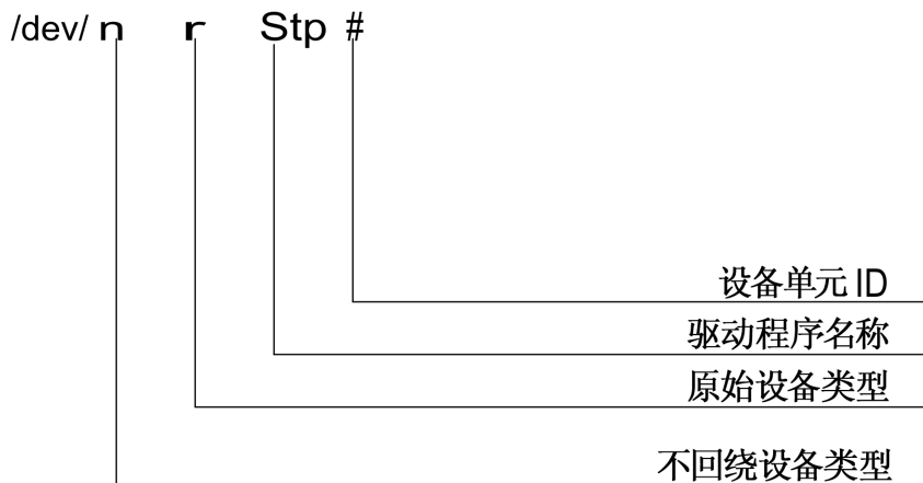
图 23 设备文件名的格式
