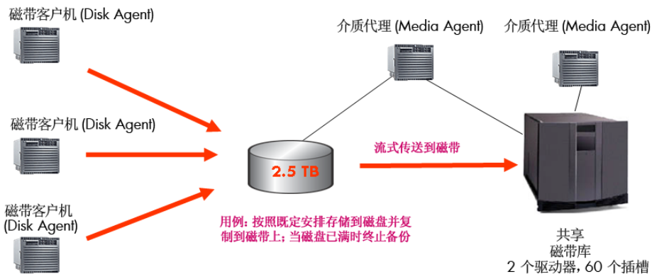
图 62 高级备份到磁盘
