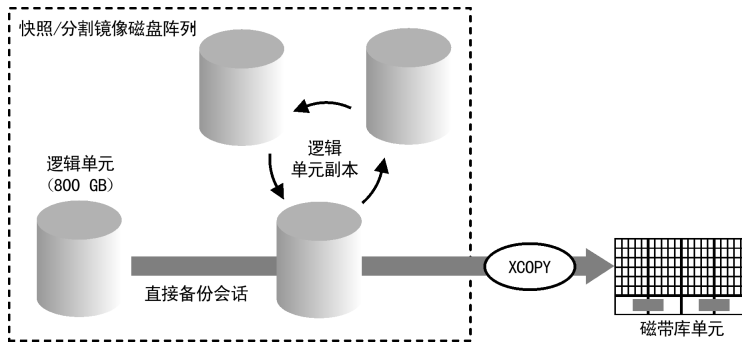
图 53 直接备份会话
