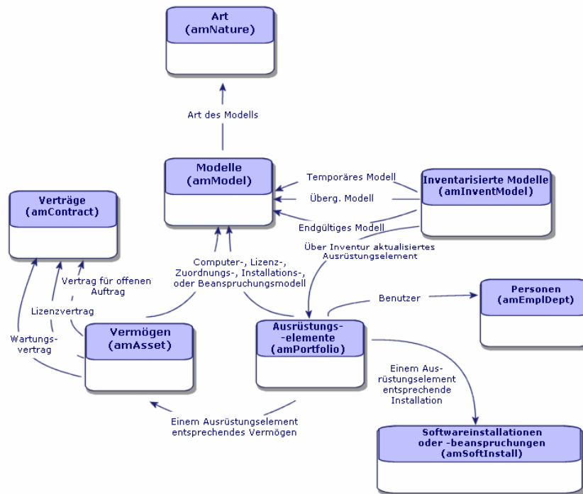
Abbildung 2.1. Physisches Datenmodell
