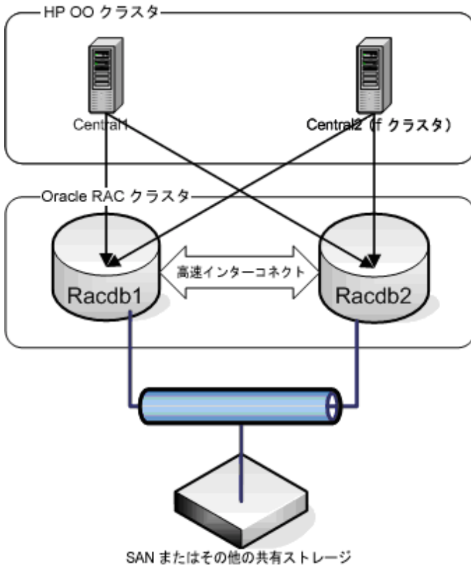
図 1 – RAC 構成の例
