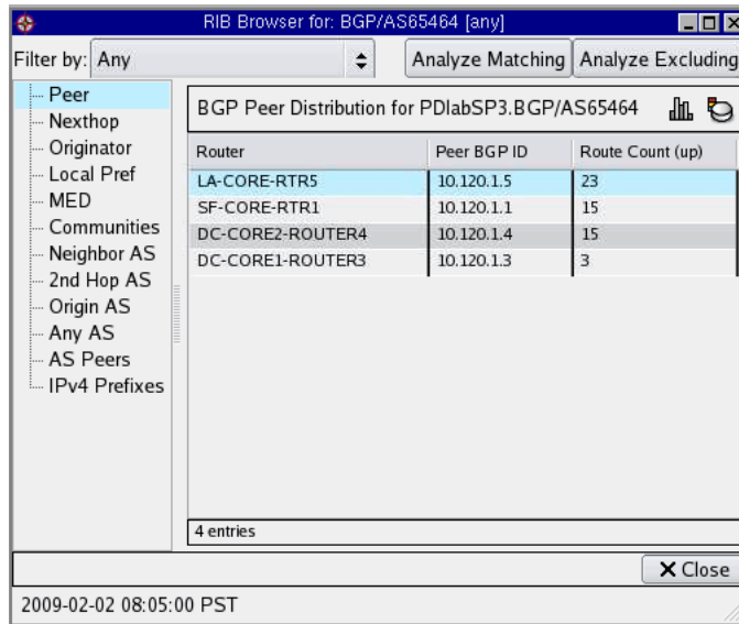
Figure 71 RIB Browser
