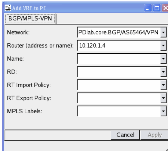
Figure 103 Add VRF to PE
