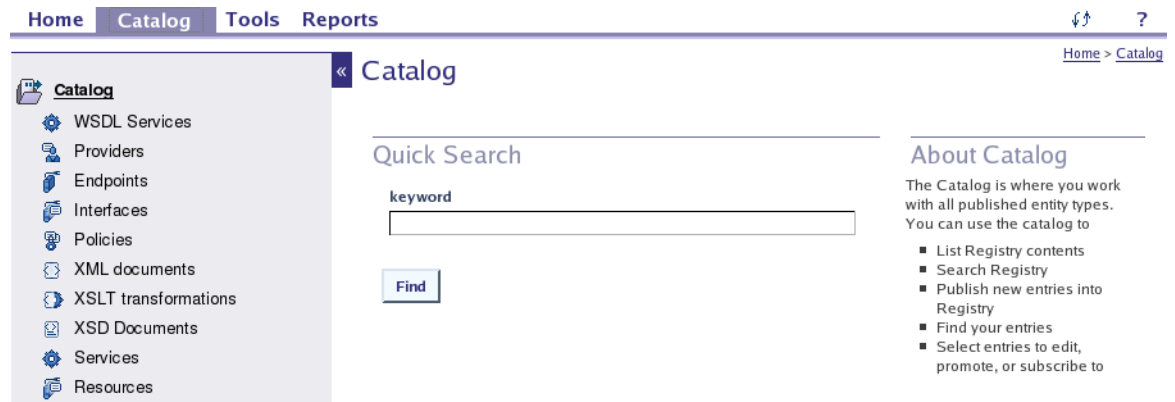
Figure 83. Catalog tab
