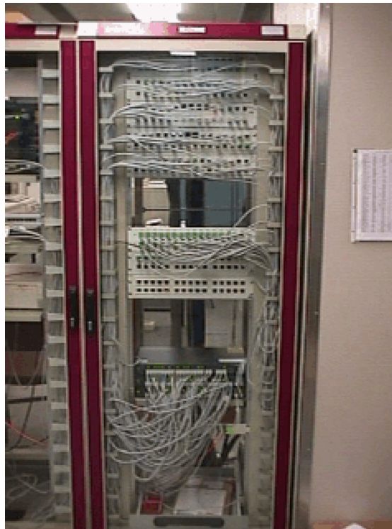
Figure 8.7. Armoire de brassage - photo
