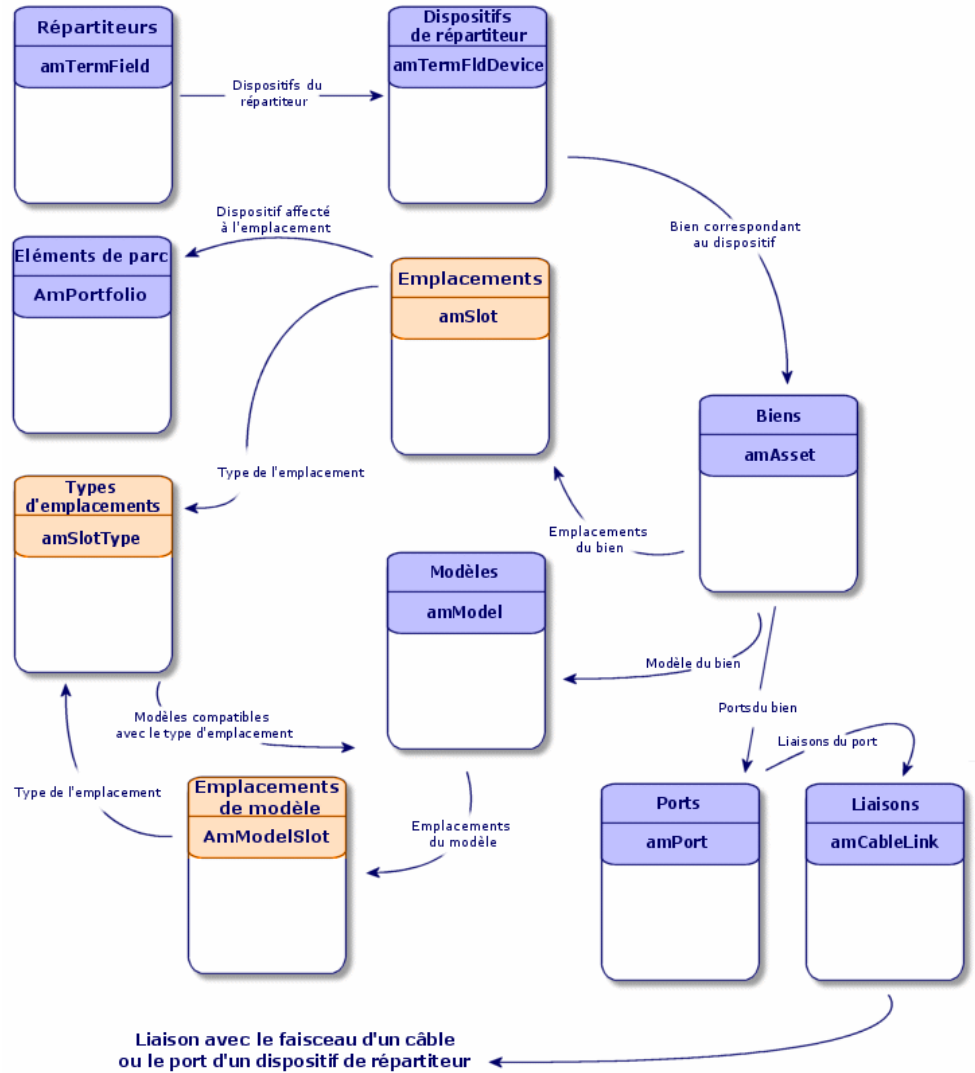
Figure 3.8. Emplacements - modèle de données
