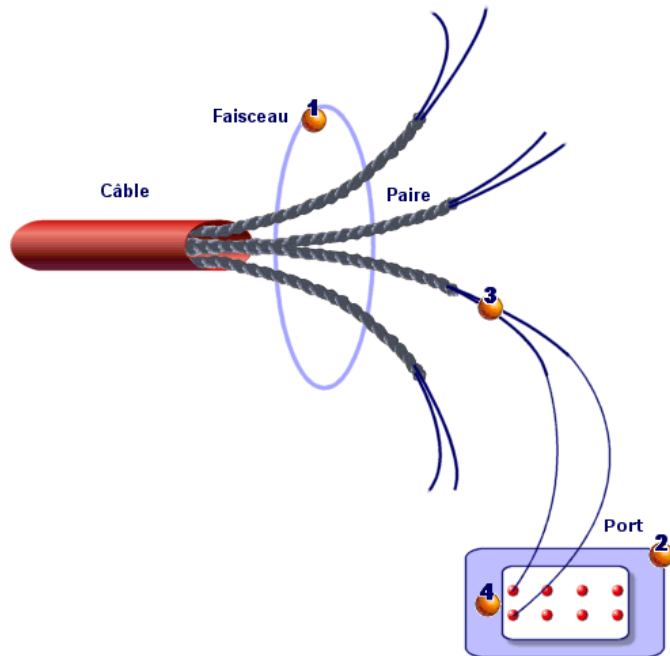
Figure 5.6. Liaison - représentation des composants impliqués
