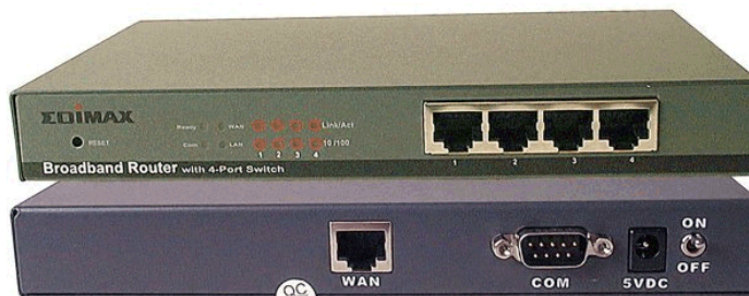
Figure 8.15. Routeur - photo
