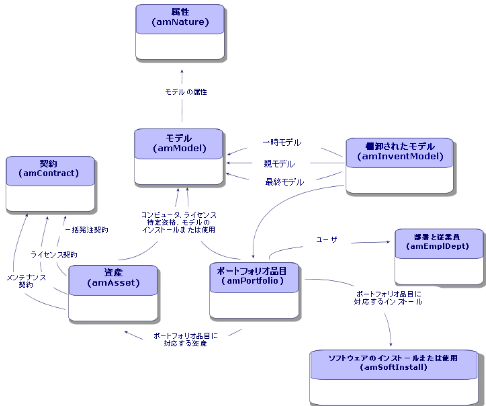
図 2.1. 物理データモデル
