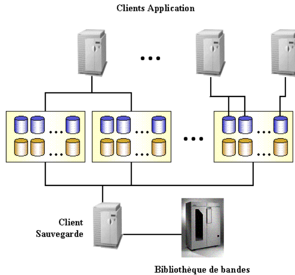
Figure 13-4 Hôtes d'application multiples - hôte de sauvegarde simple
