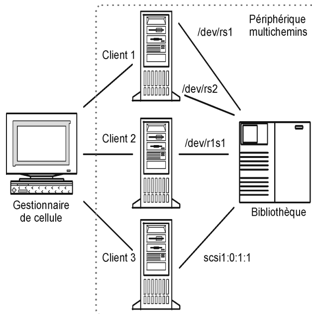
Figure 3-18 Exemple de configuration multichemins
