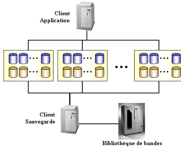
Figure 13-3 Baies de disques multiples - hôte double
