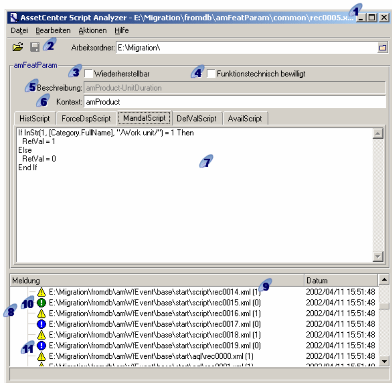
Abbildung 4.3. AssetCenter Script Analyzer - Fenster bei der Analyse von * .xml-Dateien
