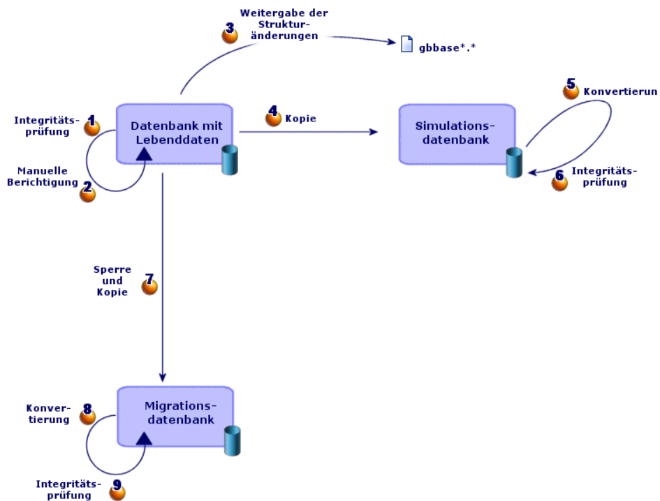
Abbildung 2.2. Konvertierung - Prozess für die AssetCenter-Version 4.2.x, 4.3.x oder 4.4.x
