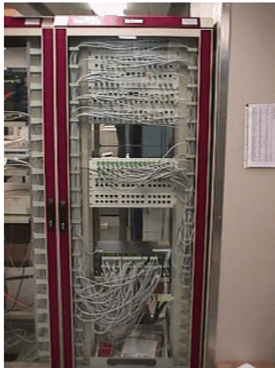
Abbildung 8.7. Steckschrank - Foto
