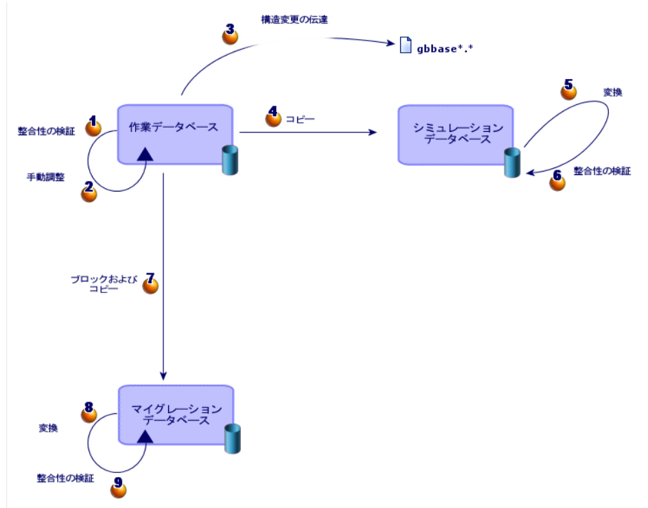
図 2.2. 変換 - AssetCenterバージョン4.2.xと4.3.xを変換するプロセス
