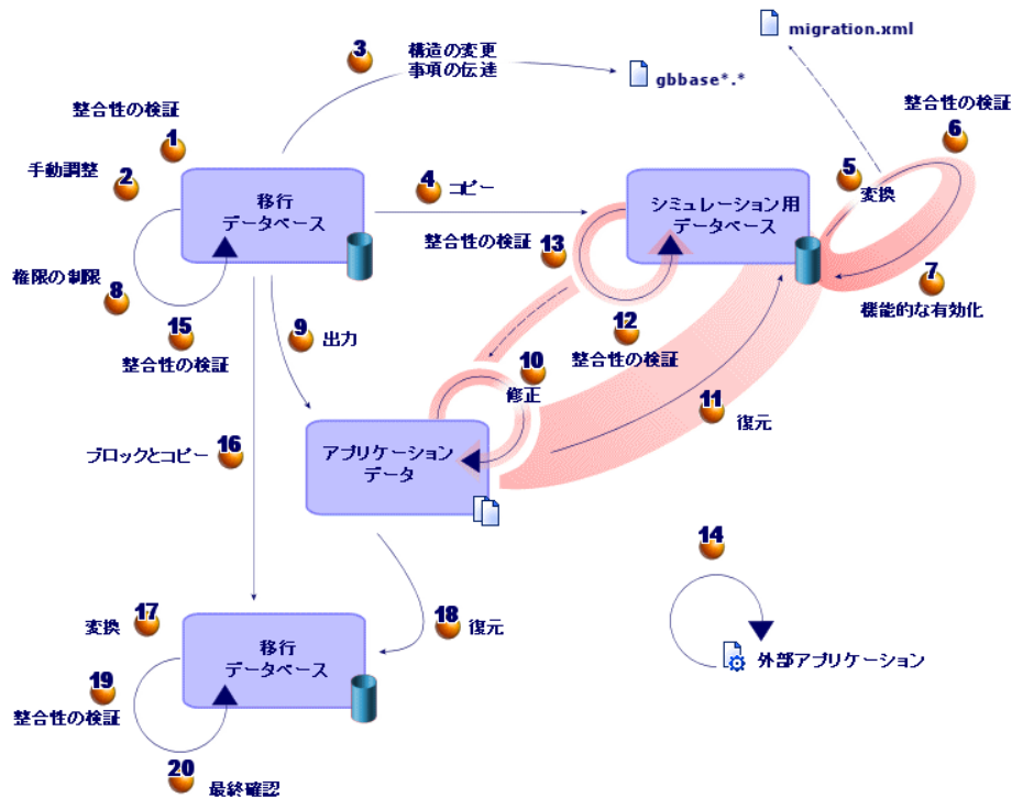
図 2.1. 変換 - AssetCenterバージョン4.1.xまたはそれ以前を変換するプロセス
