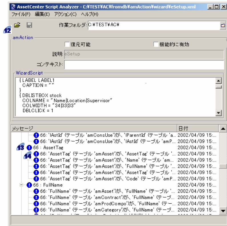
図 4.4. AssetCenter Script Analyzer - スクリプトの分析用ウィンドウ
