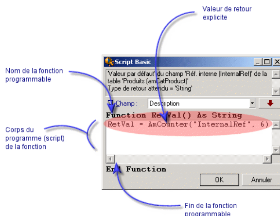
Figure 11.1. Script - constructeur
