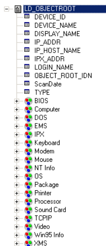
Figure 6.3. Connecteur Intel LANDesk - type de document COMPUTER_SYSTEM
