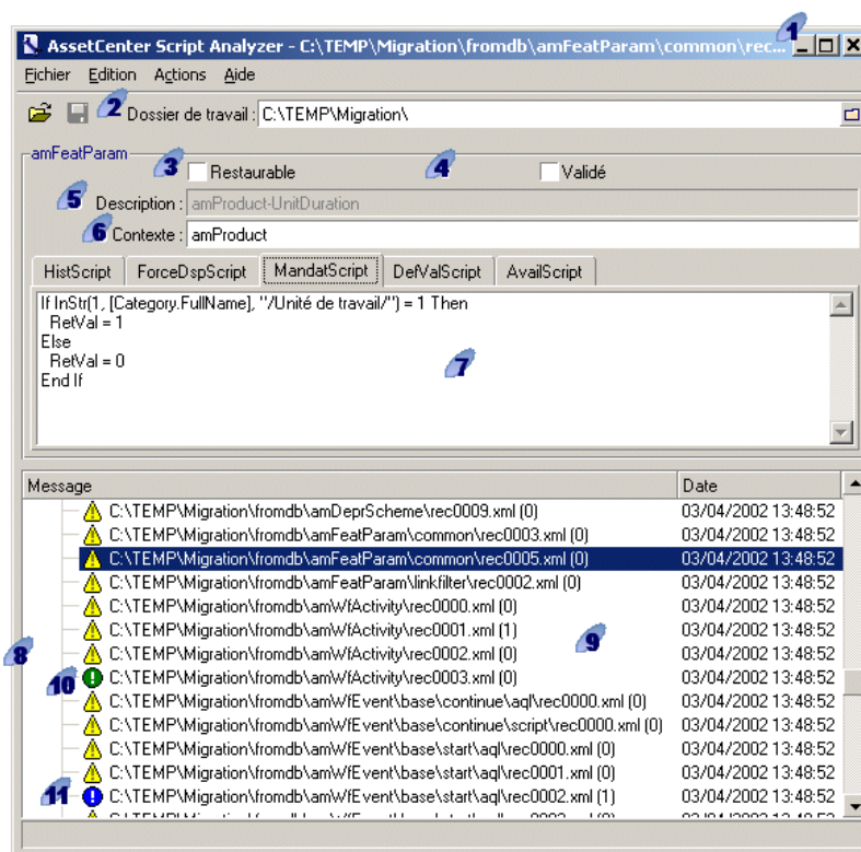
Figure 4.3. AssetCenter Script Analyzer - fenêtre d'analyse des fichiers *.xml
