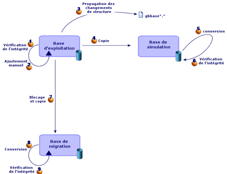
Figure 2.2. Conversion - processus pour convertir une version 4.2.x ou 4.3.x de AssetCenter
