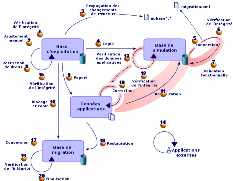
Figure 2.1. Conversion - processus pour convertir une version 4.1.x ou antérieure de AssetCenter
