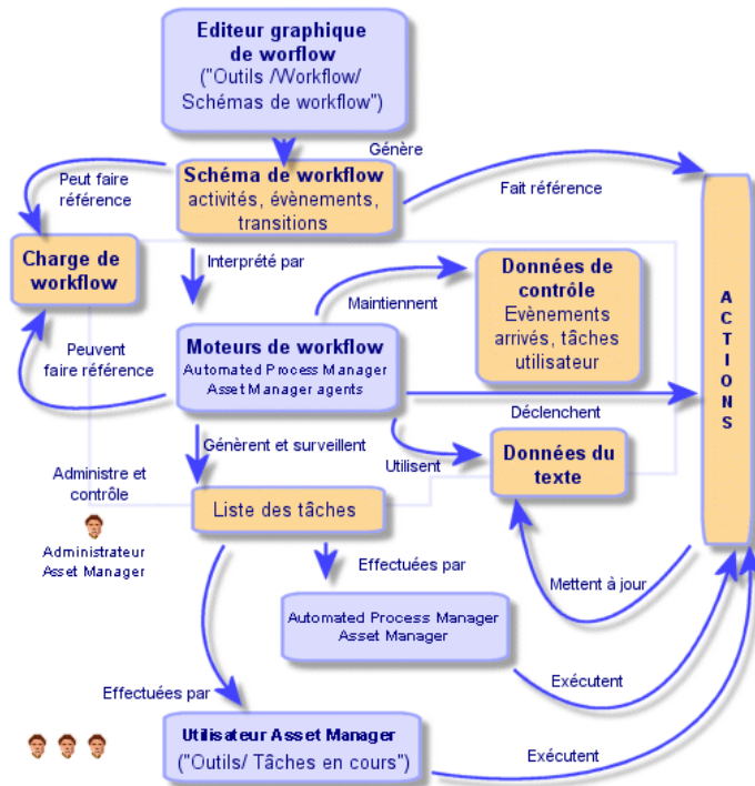
Figure 8.2. Workflow dans Asset Manager - principes généraux
