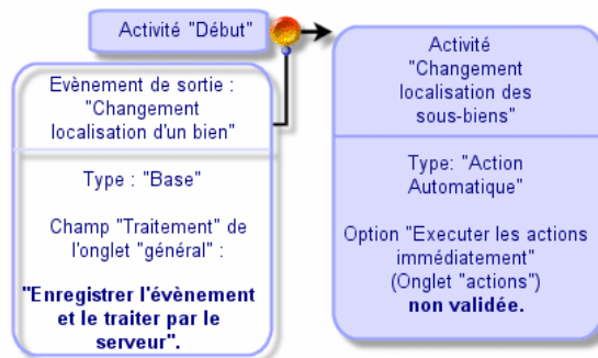
Figure 8.7. Exemple de workflow asynchrone
