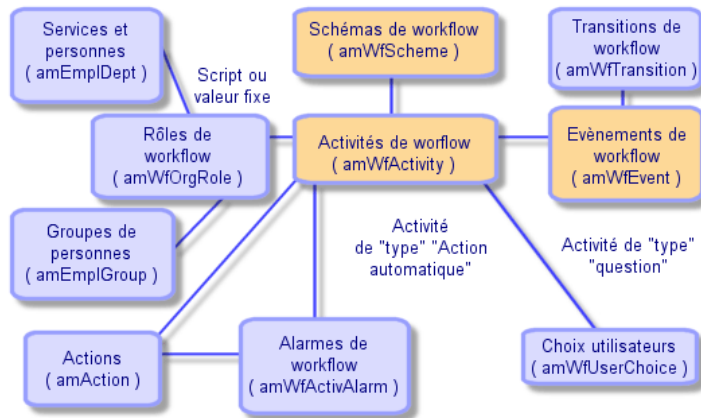
Figure 8.9. Workflow - principales tables permettant de définir un schéma
