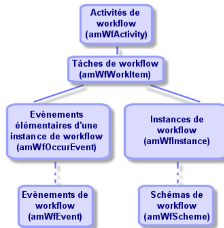
Figure 8.10. Workflow - principales tables intervenant lors du déroulement d'une instance
