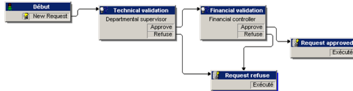
Figure 8.4. Workflow - schéma de validation des demandes
