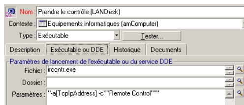
Figure 7.1. Action de type exécutable - fenêtre de détail
