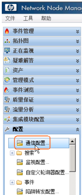
图 6：通信配置
