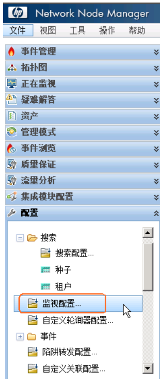
图 25: 监视配置
