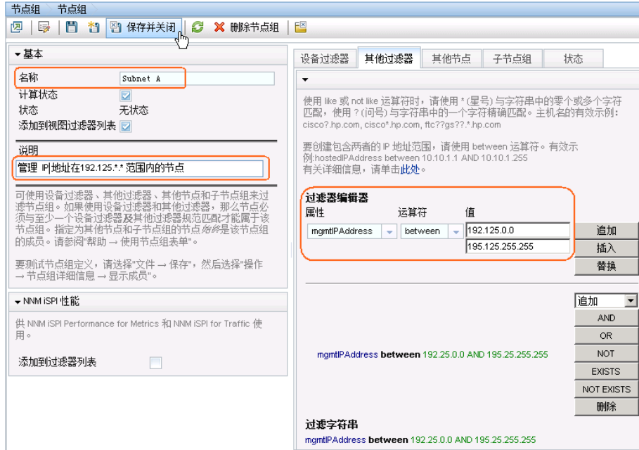
图 45：节点组：基本
