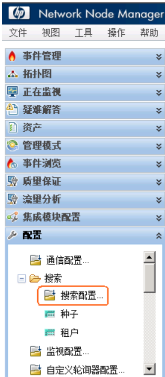
图 10: 搜索配置
