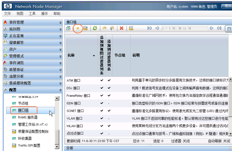
图 21: 配置: 接口组
