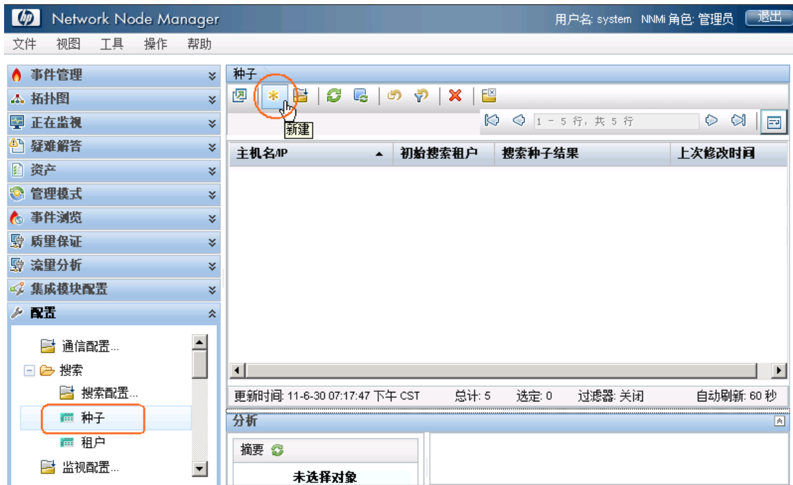
图 14：搜索：种子
