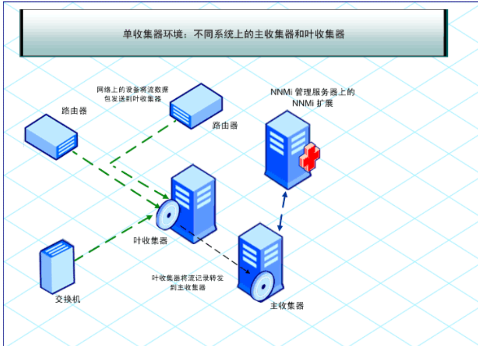
图 4 两个收集器在同一个系统上
