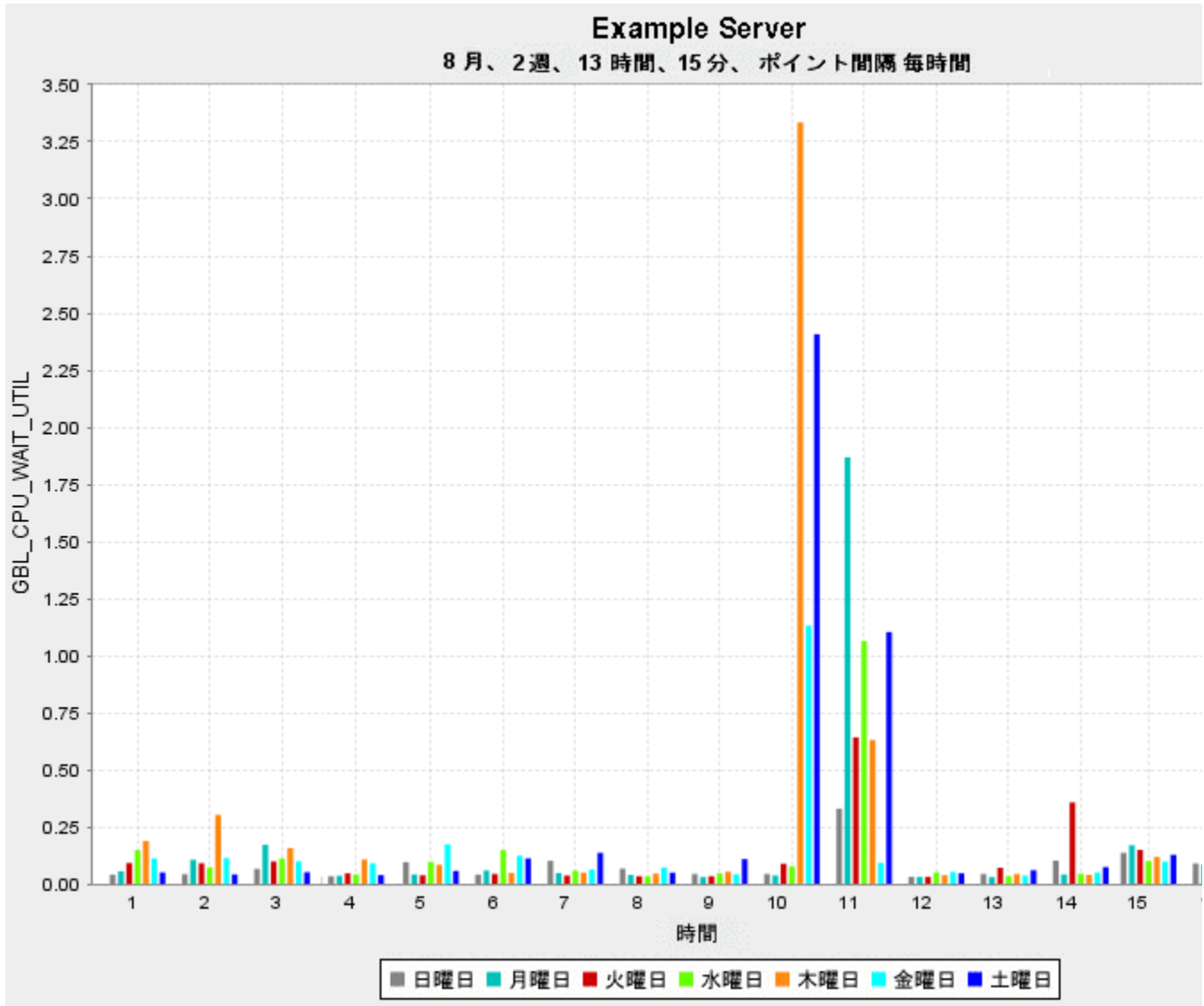
図5 使用率が低いシステムのデータを使用した CPU 使用率グラフの例
