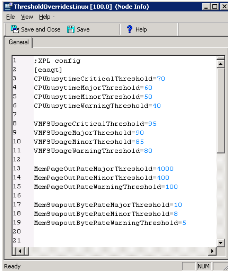
図4 しきい値の無効化ポリシーの例
