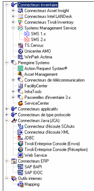
Figure 5.1. Boîte à outils de l'éditeur de scénarios
