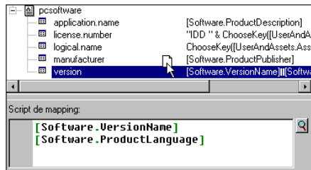
Figure 7.1. Glisser-déplacer plusieurs champs
