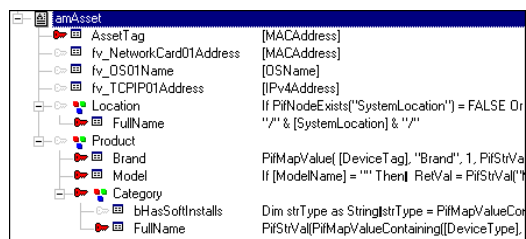
Figure 6.2. Résumé des scripts de mapping sur le plan de travail
