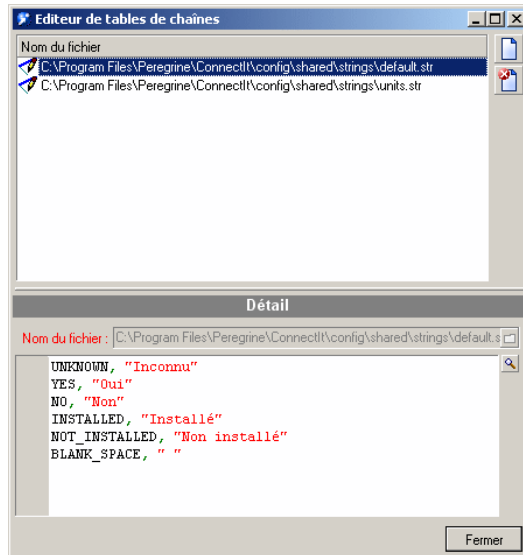
Figure 7.2. L'éditeur des tables de correspondance
