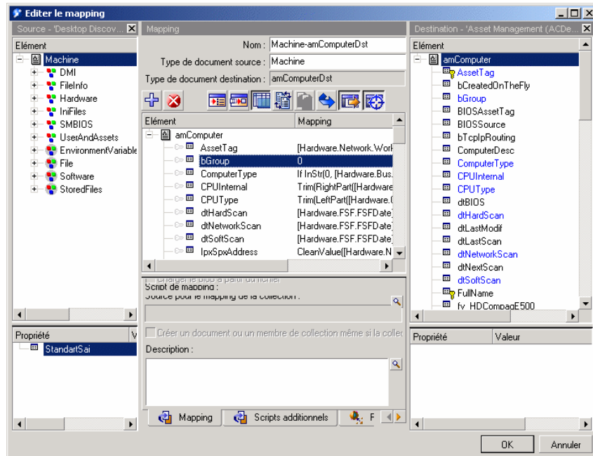
Figure 6.1. Fenêtre d'édition d'un mapping
