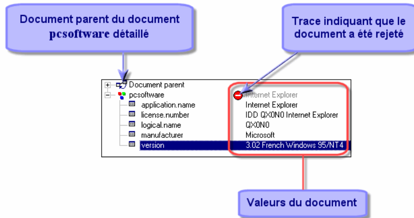
Figure 3.9. Détail du document pcsoftware consommé par le connecteur ServiceCenter
