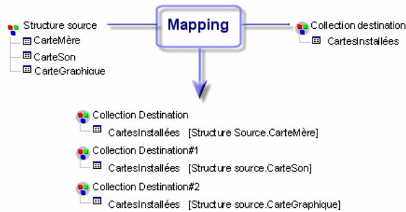
Figure 6.7. Mapping champ à collection
