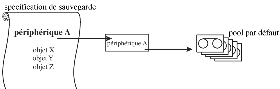
Figure 39 Relation simple entre un périphérique et un pool de supports
