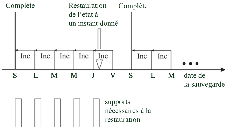
Figure 30 Sauvegarde complète avec des sauvegardes incrémentales simples quotidiennes
