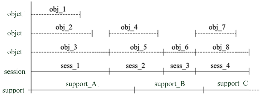
Figure 44 Plusieurs objets et sessions par support, écritures simultanées
