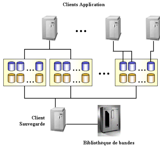
Figure 80 Hôtes d'application multiples - hôte de sauvegarde simple
