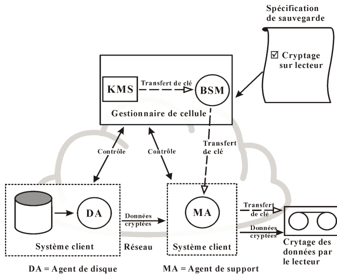
Figure 18 Session de sauvegarde avec cryptage AES 256 bits et cryptage sur lecteur
