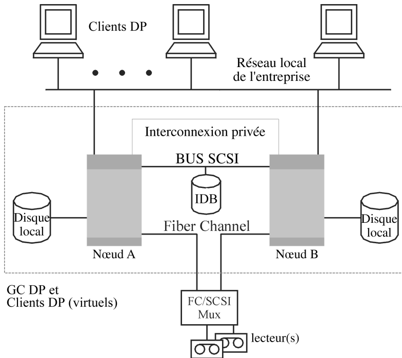
Figure 24 Gestionnaire de cellule installé dans un cluster, périphériques connectés aux nœuds de cluster
