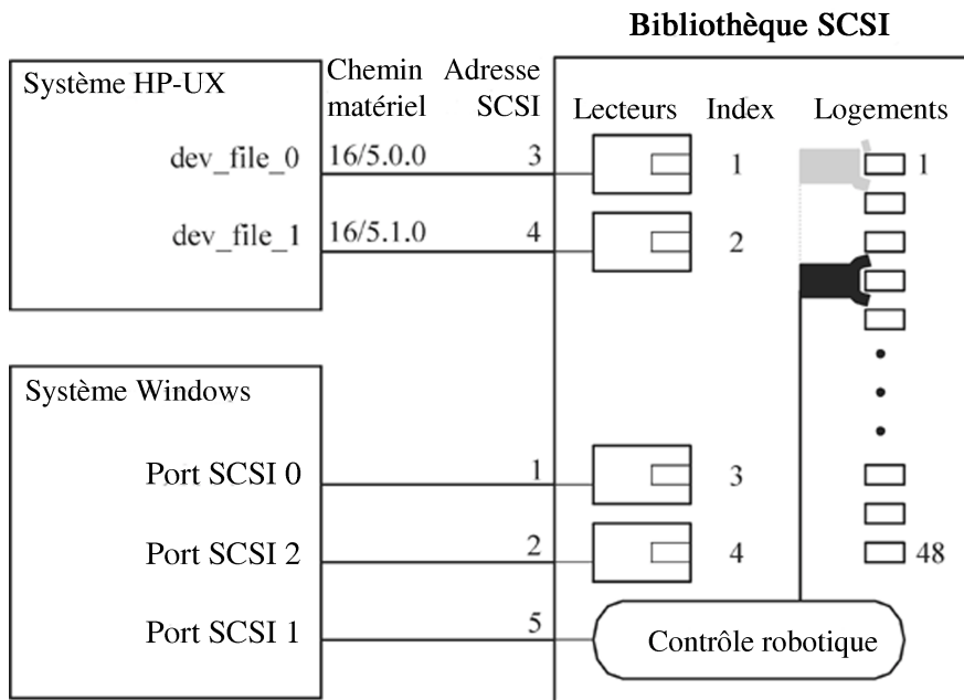
Figure 49 Connexion de lecteurs à plusieurs systèmes
