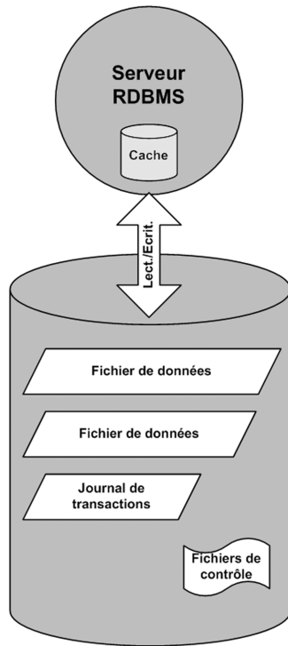
Figure 65 Base de données relationnelle
