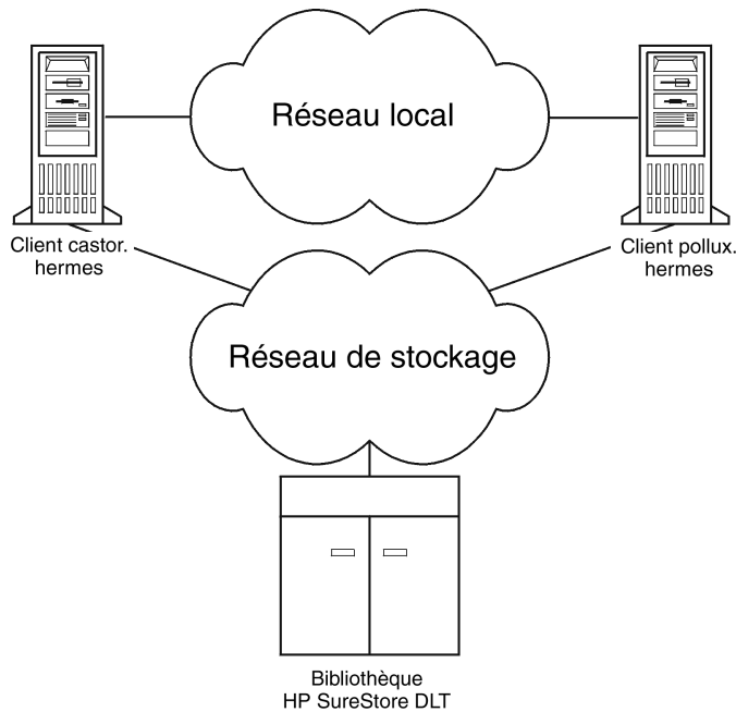
Figure 57 Accès direct à la bibliothèque
