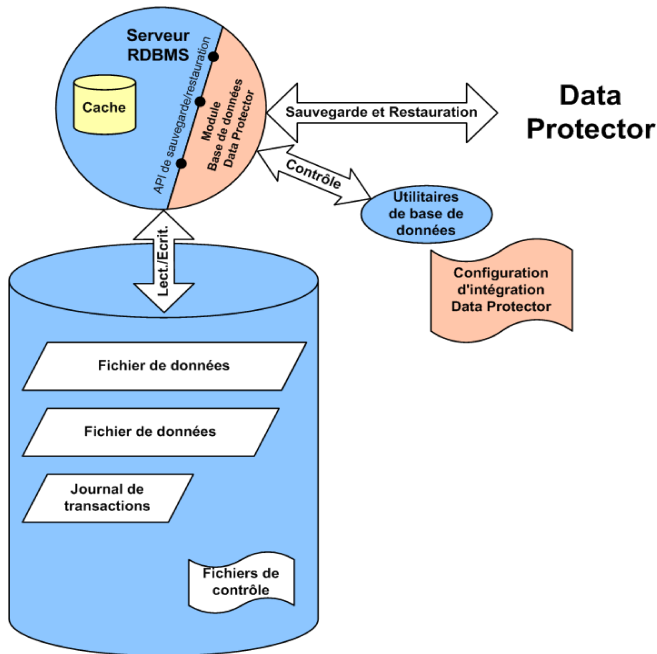
Figure 66 Intégration de Data Protector à des bases de données
