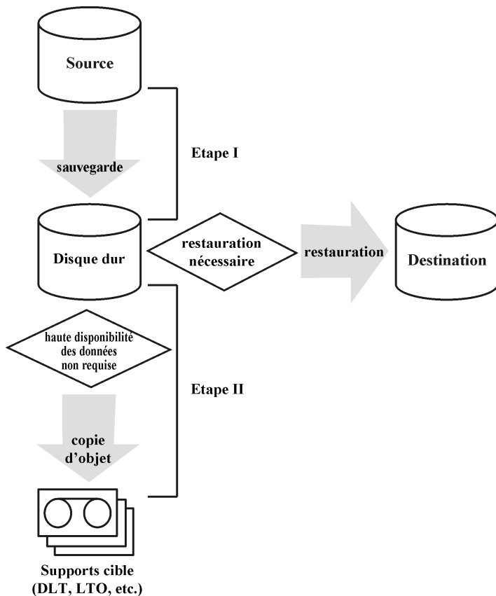
Figure 36 Concept de sauvegarde de disque en plusieurs étapes
