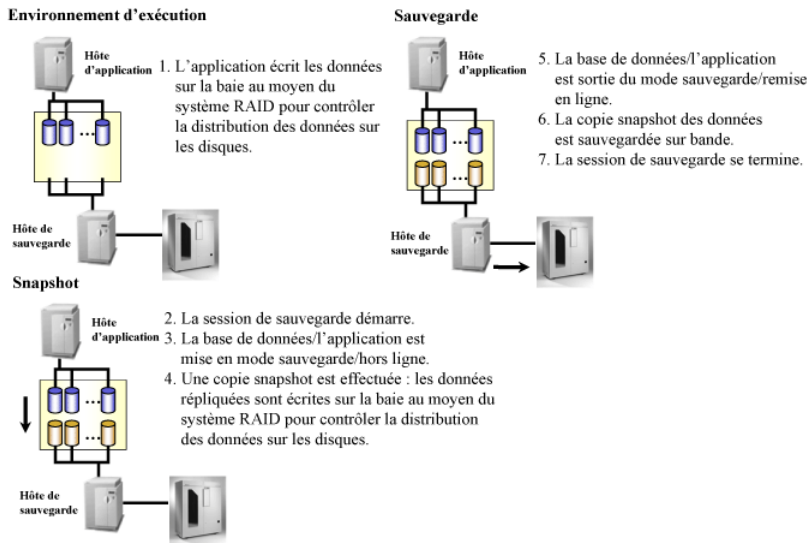
Figure 77 Sauvegarde de snapshot
