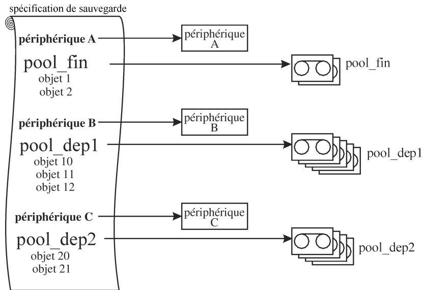
Figure 40 Configuration des pools de supports pour les grandes bibliothèques
