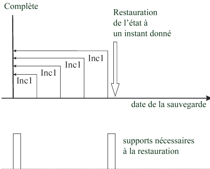
Figure 28 Supports nécessaires à la restauration à partir de sauvegardes incrémentales par niveau
