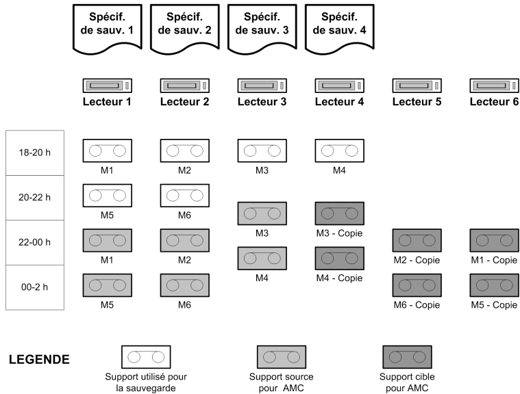
Figure 94 Sauvegarde Incr1 et copie automatisée de supports
