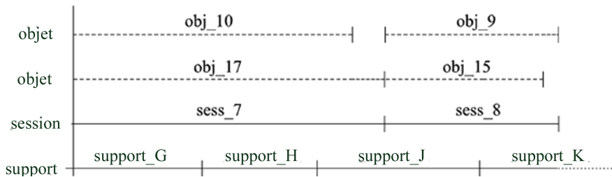
Figure 45 Plusieurs supports par session et par objet
