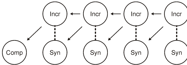
Figure 71 Sauvegarde synthétique régulière
