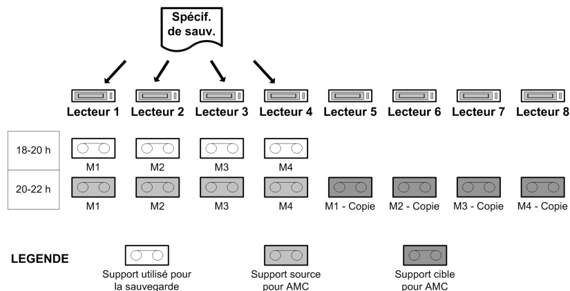
Figure 97 Sauvegarde complète de base de données et copie automatisée de supports
