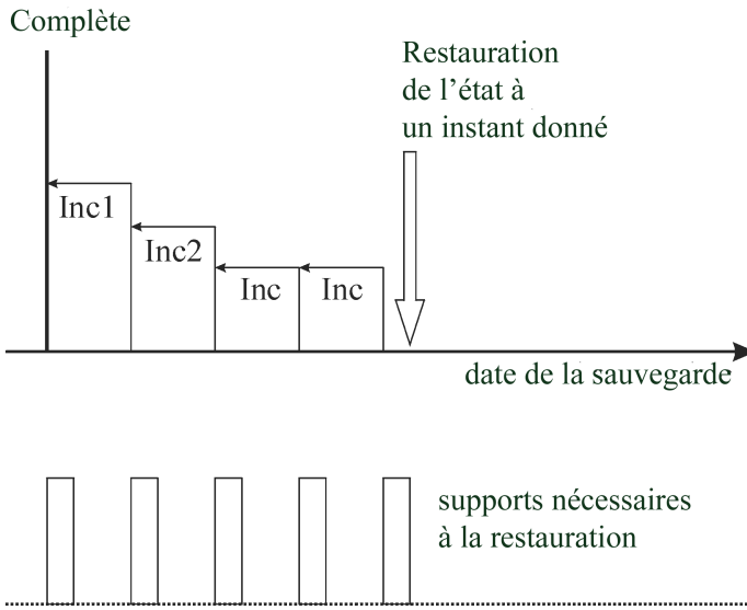
Figure 27 Supports nécessaires à la restauration à partir de sauvegardes incrémentales simples et par niveau
