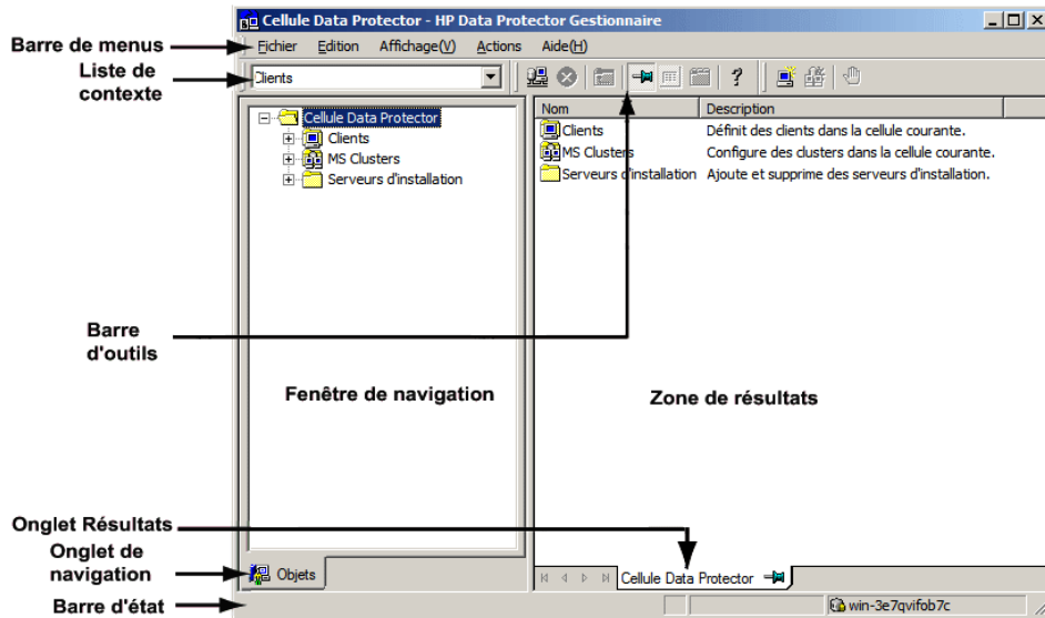
Figure 14 Interface graphique Data Protector d'origine
