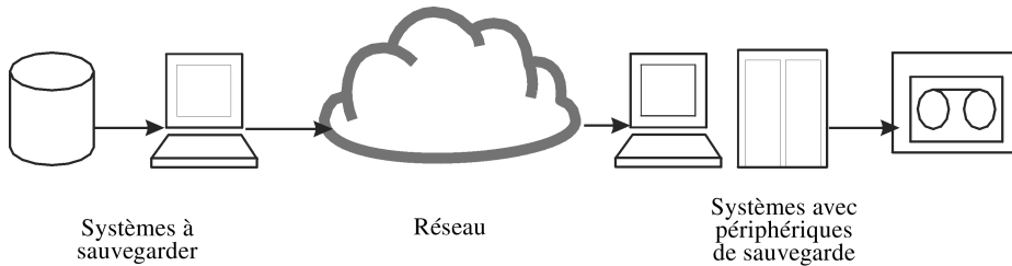
Figure 4 Sauvegarde réseau
