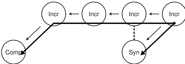
Figure 70 Sauvegarde synthétique
