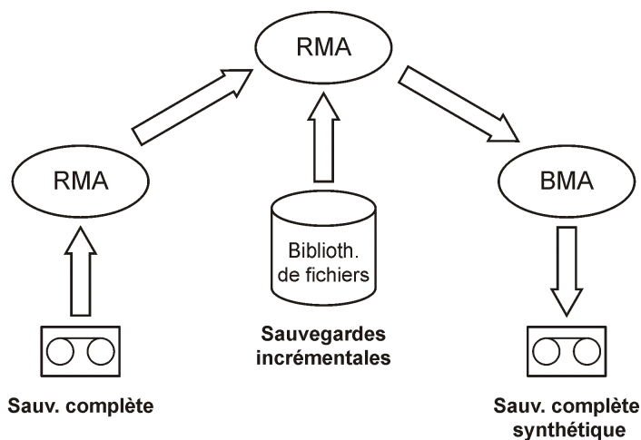
Figure 67 Sauvegarde synthétique
