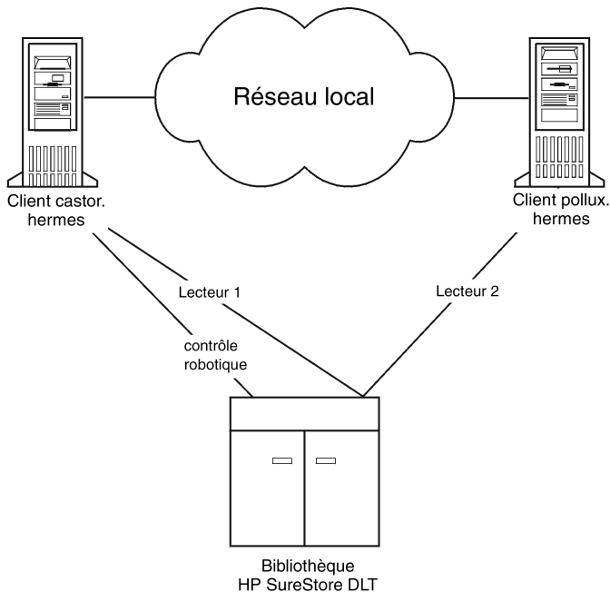
Figure 56 Accès indirect à la bibliothèque
