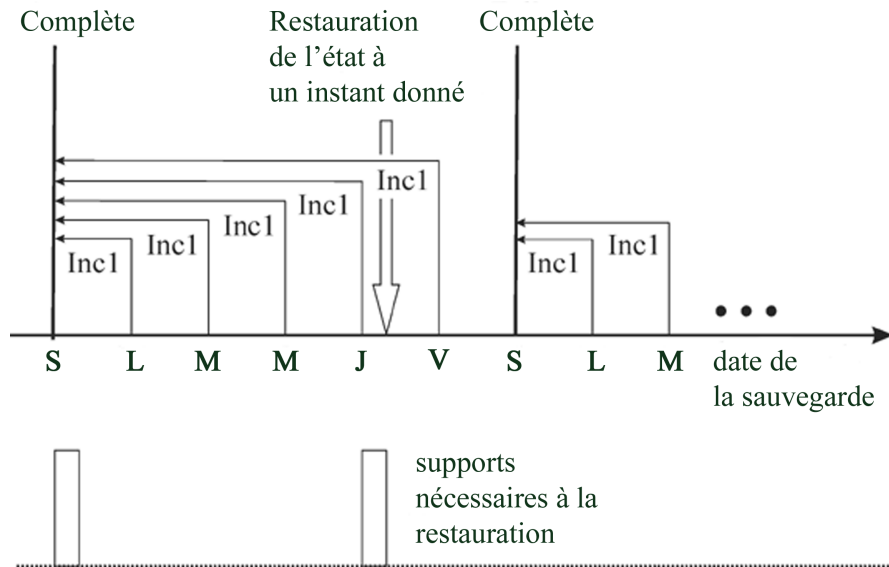
Figure 31 Sauvegarde complète avec des sauvegardes incrémentales quotidiennes de niveau 1
