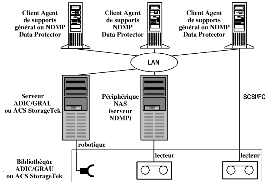
Figure 52 Partage d'une bibliothèque ADIC/GRAU ou StorageTek ACS
