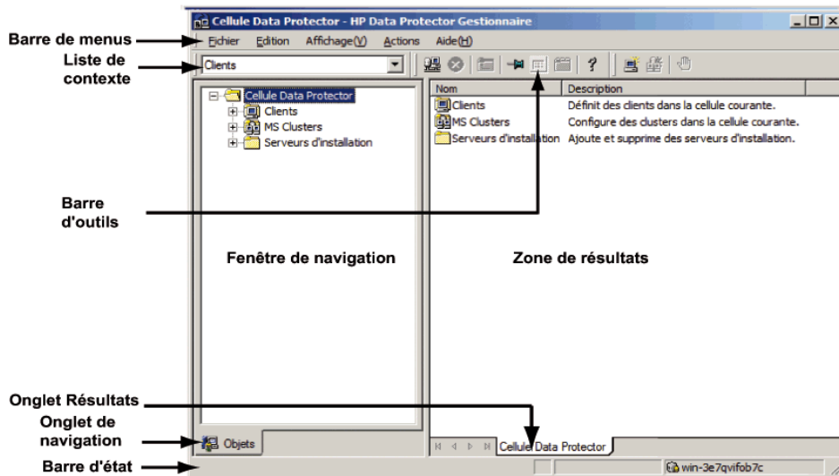
Figure 15 interface graphique Java de Data Protector
