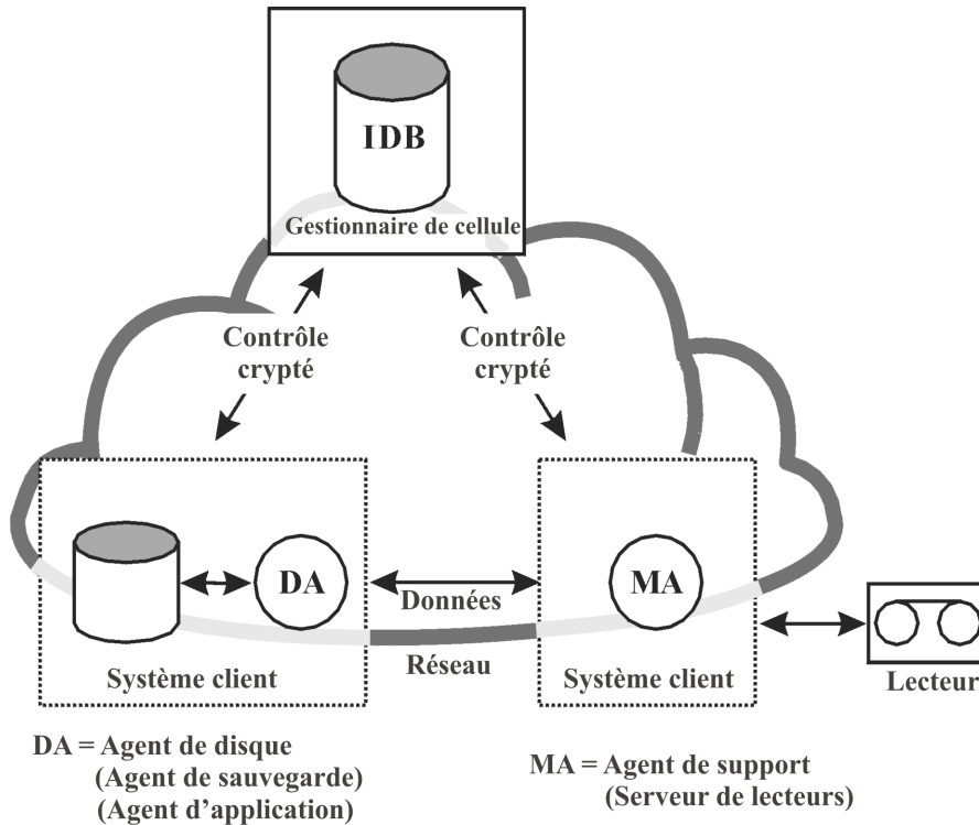
Figure 19 Communications de contrôle cryptées
