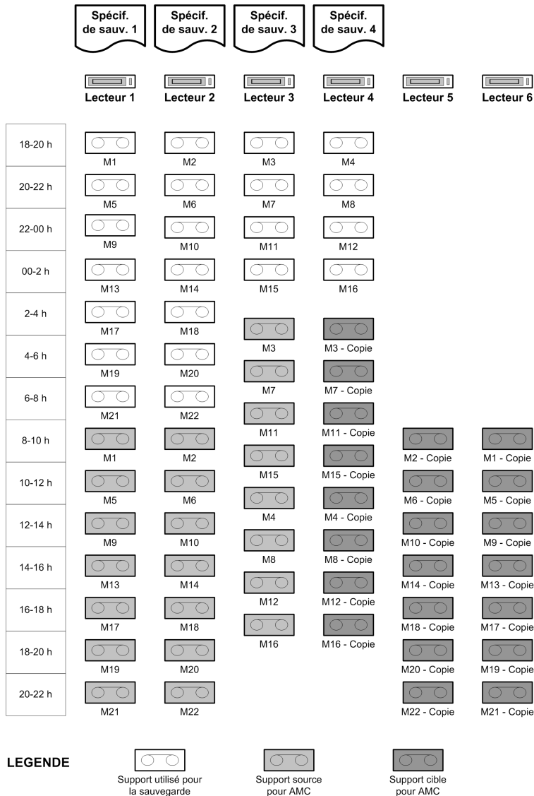
Figure 95 Sauvegarde complète et copie automatisée de supports
