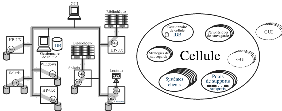
Figure 5 Cellule Data Protector (description physique et logique)
