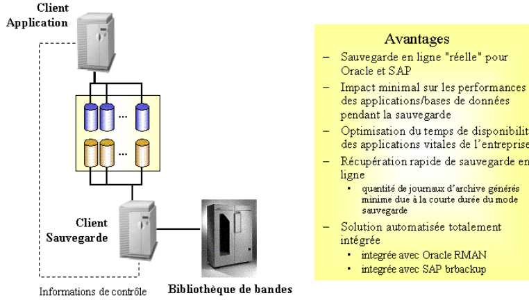
Figure 78 Baie de disques simple - hôte double (sauvegarde avec performance optimale et temps d'indisponibilité nul)
