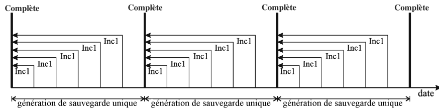
Figure 93 Générations de sauvegarde
