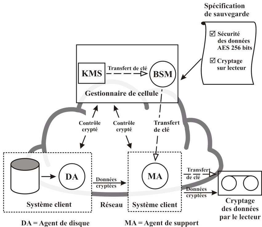
Figure 20 Communications de contrôle cryptées et cryptage des données
