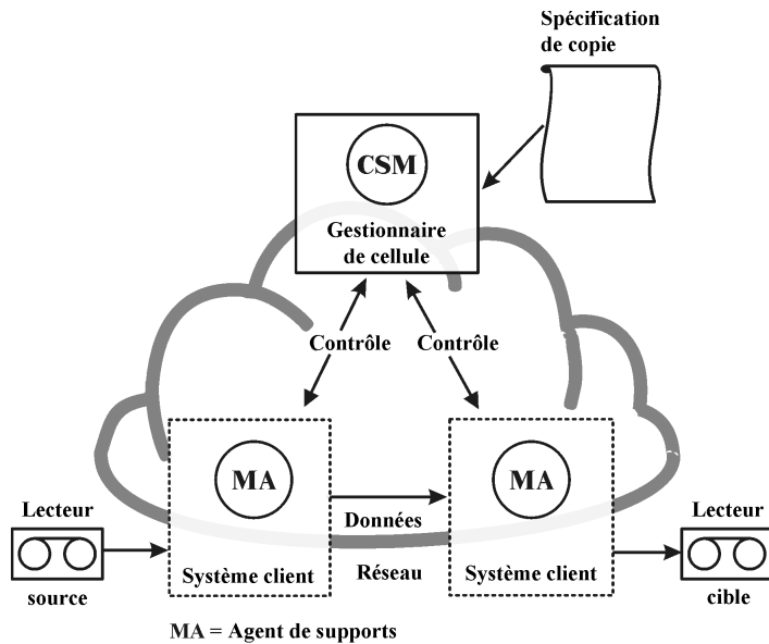
Figure 64 Flux de données d'une session de copie d'objet
