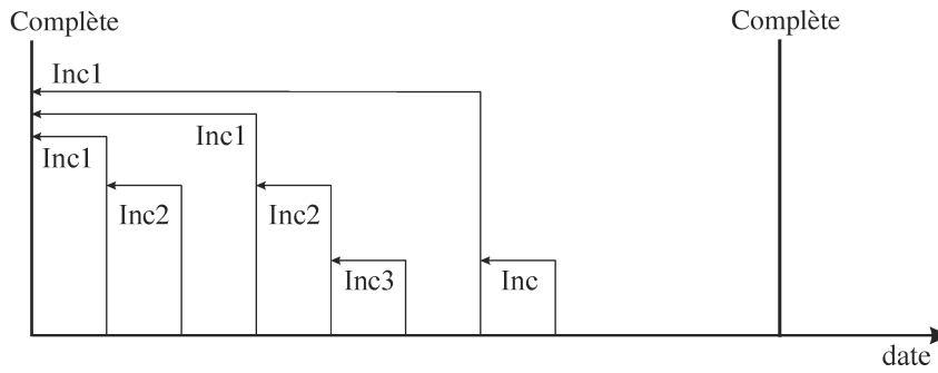
Figure 26 Sauvegardes incrémentales par niveau
