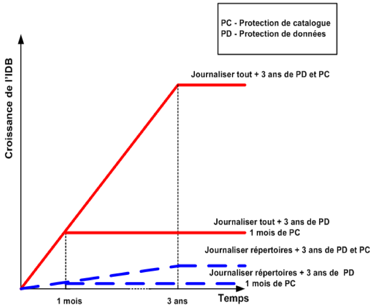
Figure 59 Influence du niveau de journalisation et de la protection de catalogue sur la croissance de la base de données IDB
