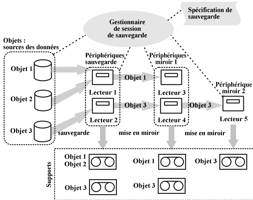
Figure 37 Mise en miroir d'objets
