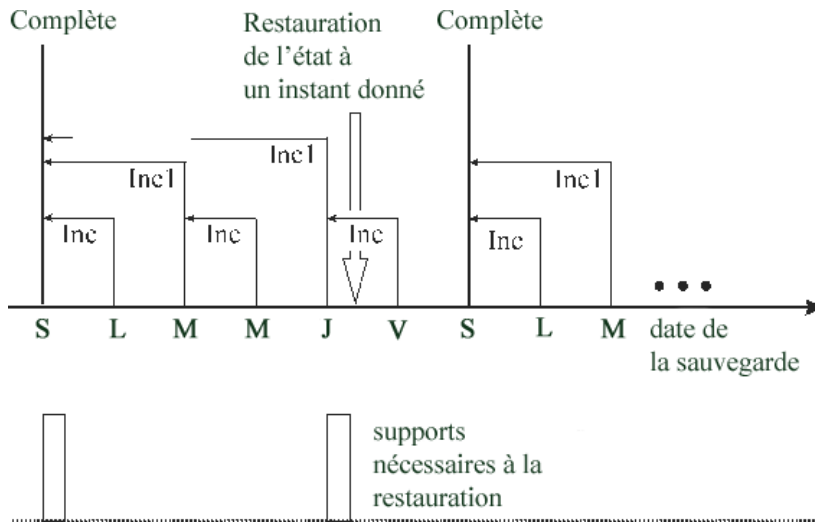
Figure 32 Sauvegarde complète avec des sauvegardes incrémentales mixtes
