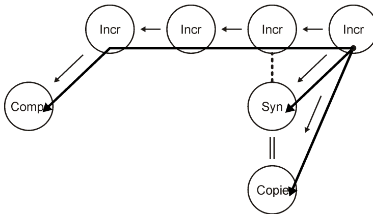
Figure 72 Sauvegarde synthétique et copie d'objet
