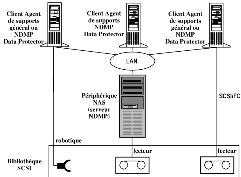
Figure 50 Partage d'une bibliothèque SCSI (robot relié à un système client Data Protector)
