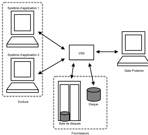
Figure 83 Acteurs du modèle de sauvegarde VSS
