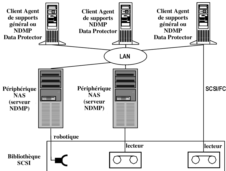
Figure 51 Partage d'une bibliothèque SCSI (robot relié à un serveur NDMP)
