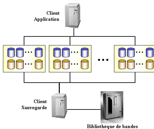
Figure 79 Baies de disques multiples - hôte double
