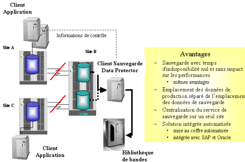
Figure 75 Split Mirror - miroir distant (sauvegarde distante indépendante du réseau local - données haute disponibilité)
