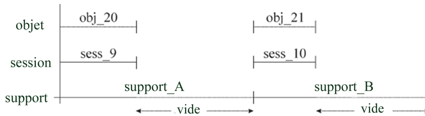
Figure 46 Chaque objet est écrit sur un support séparé
