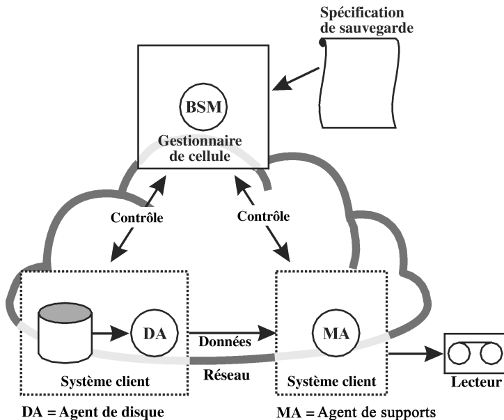
Figure 60 Flux de données de la session de sauvegarde (1)
