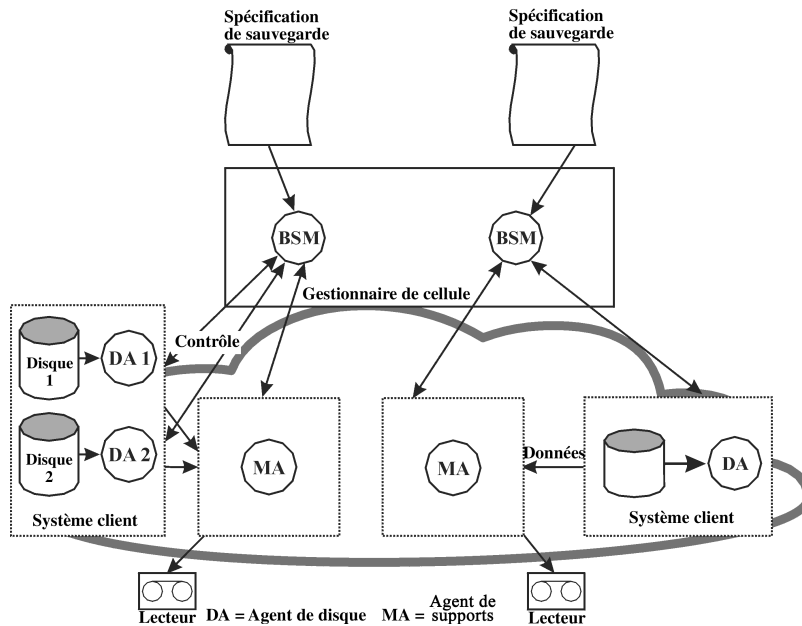
Figure 61 Flux de données d'une session de sauvegarde - sessions multiples
