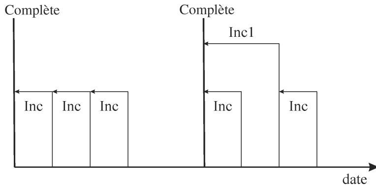
Figure 25 Sauvegardes incrémentales
