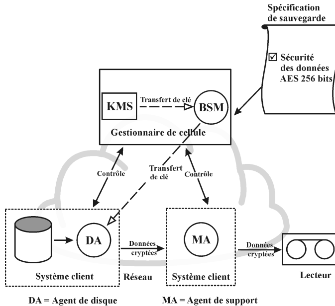
Figure 17 Session de sauvegarde avec cryptage AES 256 bits
