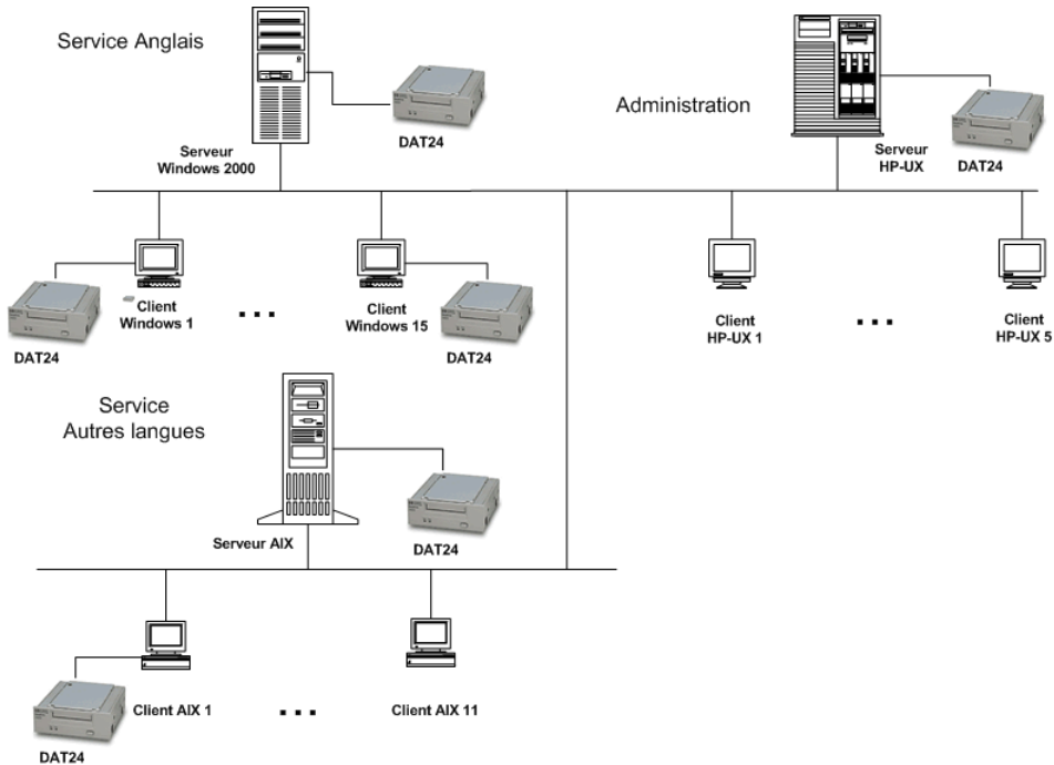
Figure 84 Topologie de sauvegarde actuelle de XYZ
