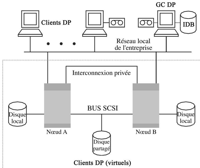
Figure 22 Gestionnaire de cellule installé hors d'un cluster
