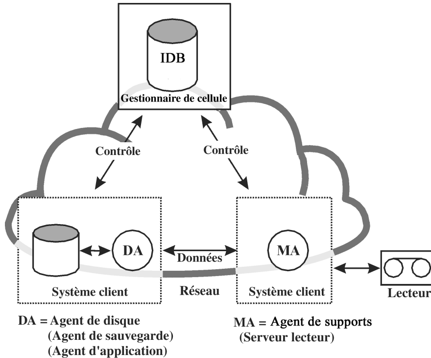
Figure 6 Opération de sauvegarde ou de restauration
