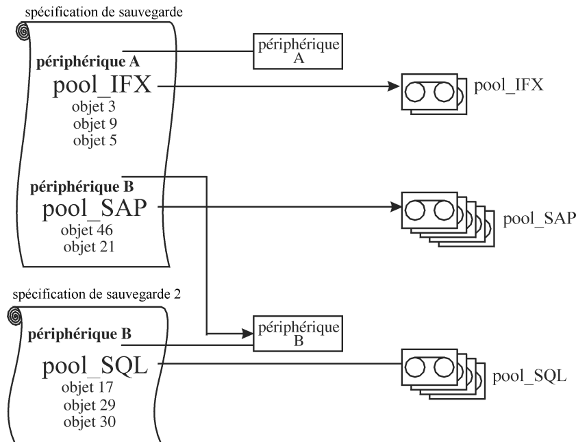
Figure 42 Périphériques multiples, pools de supports multiples
