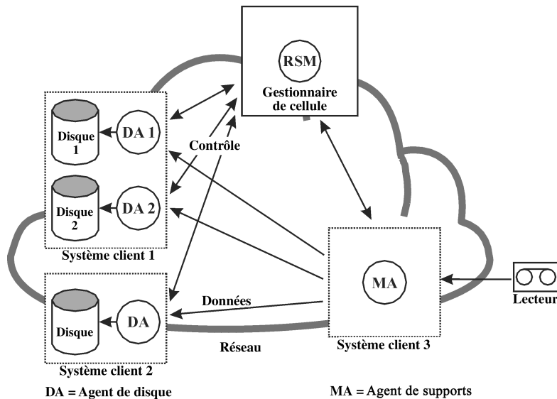
Figure 63 Flux de session d'une restauration parallèle
