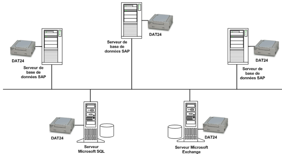
Figure 88 Topologie de sauvegarde actuelle d'ABC Le Cap
