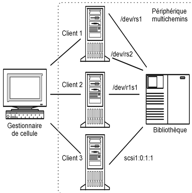
Figure 55 Exemple de configuration multichemins
