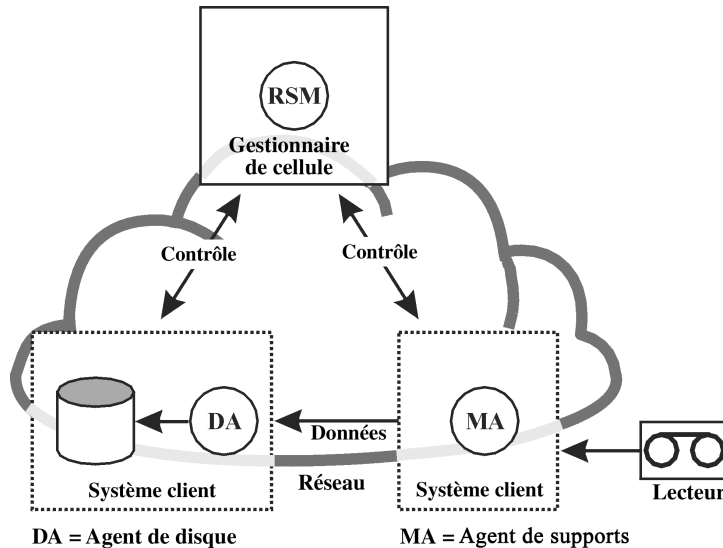
Figure 62 Flux de données d'une session de restauration
