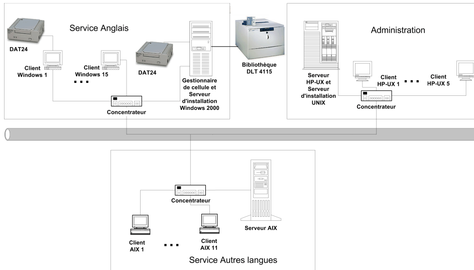
Figure 85 Topologie de sauvegarde proposée pour XYZ
