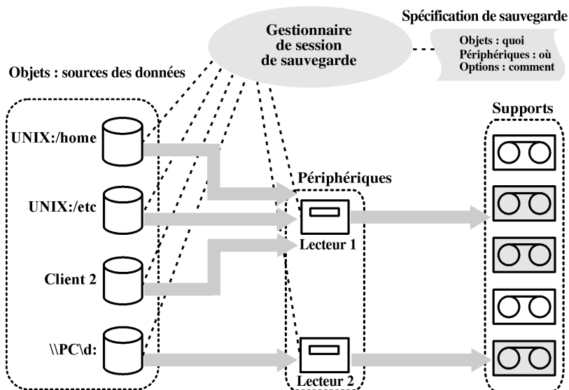
Figure 29 Session de sauvegarde
