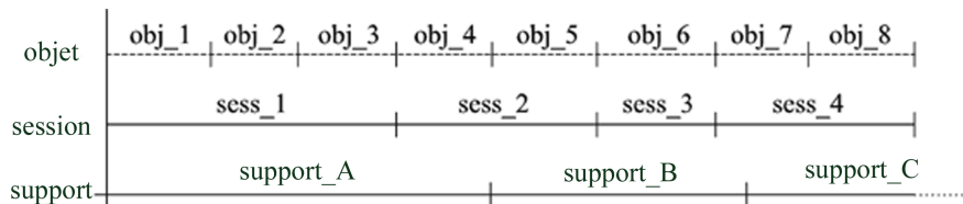
Figure 43 Plusieurs objets et sessions par support, écritures séquentielles
