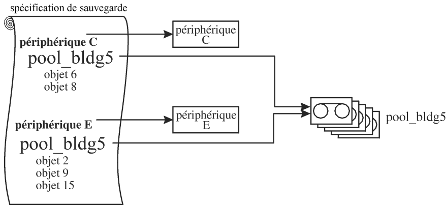
Figure 41 Périphériques multiples, pool de supports unique
