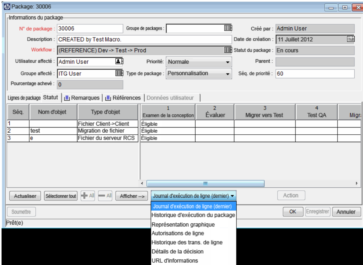
Figure 2-12. Fenêtre de package, onglet Statut
