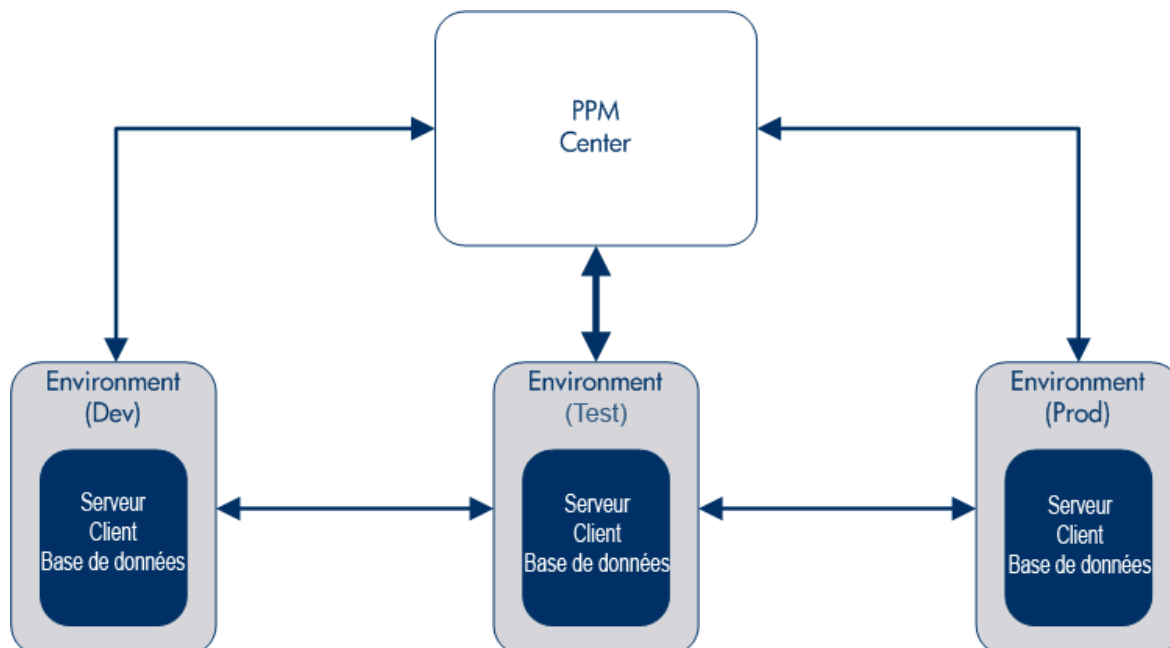
Figure 2-1. Traitement des packages dans Deployment Management
