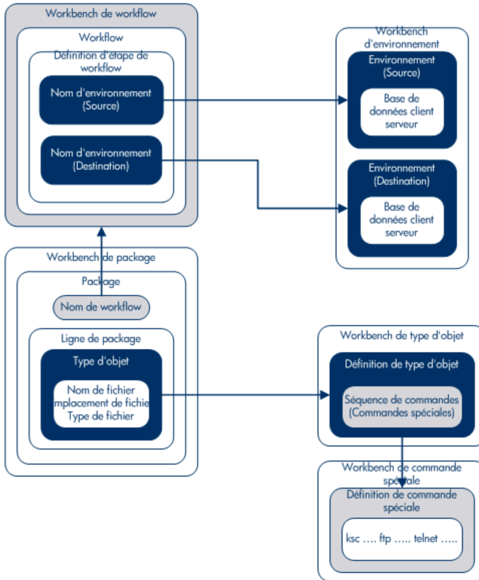
Figure 2-3. Processus de formation d'un package
