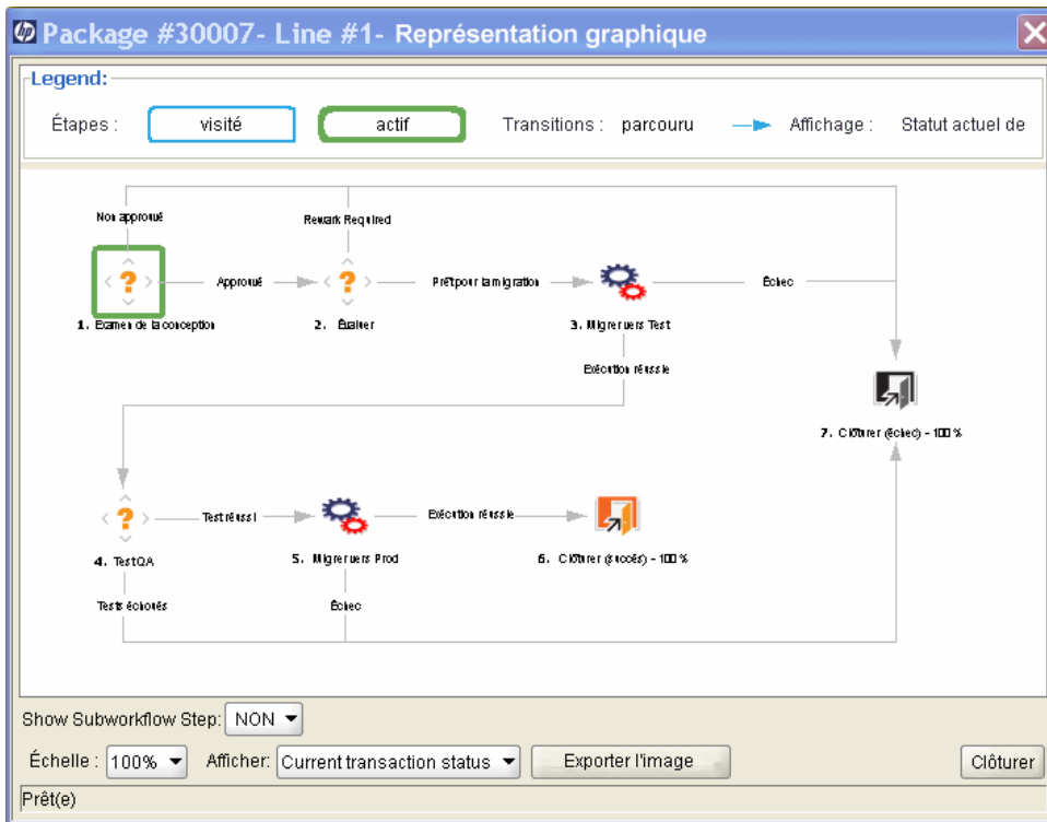
Figure 2-13. Fenêtre Représentation graphique pour un package
