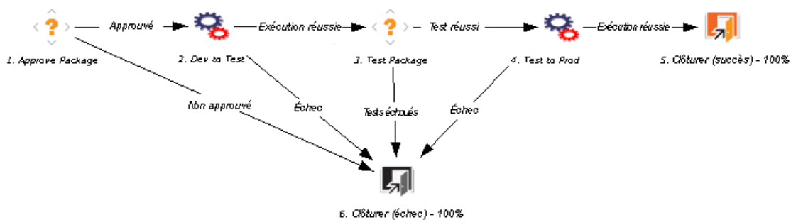
Figure 2-2. Workflow du package et étapes de workflow
