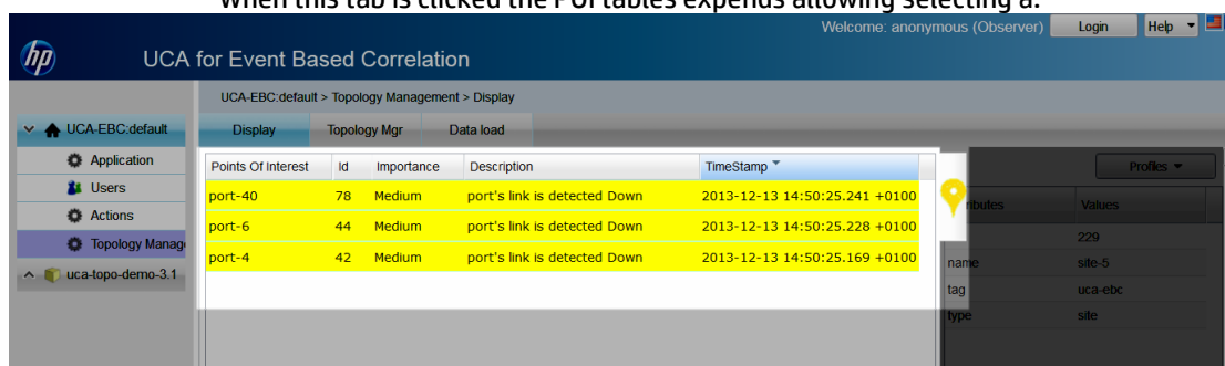
Figure 10 - POI Table
