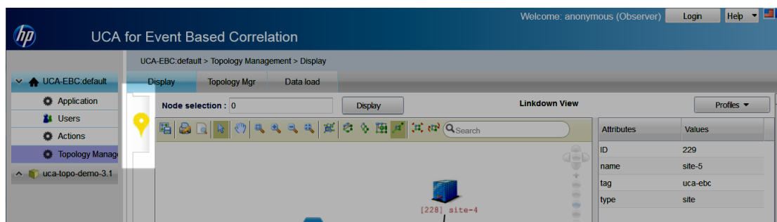
Figure 9 - POI Tab
