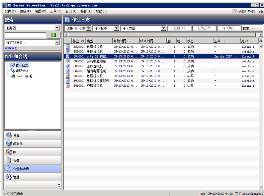
图 37.SA 作业和会话中的作业状态
