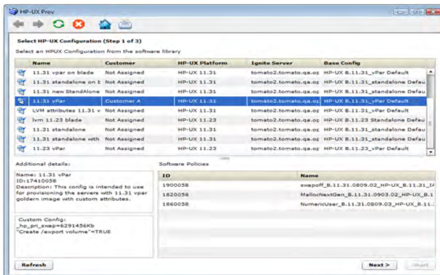
图 29. HP-UX Provisioning APX - 选择 HP-UX 配置
