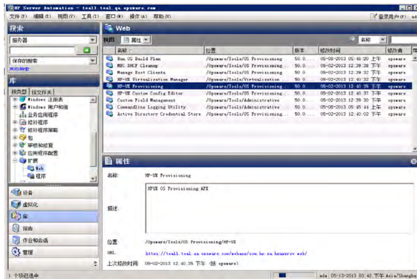
图 27.HP-UX Provisioning APX
