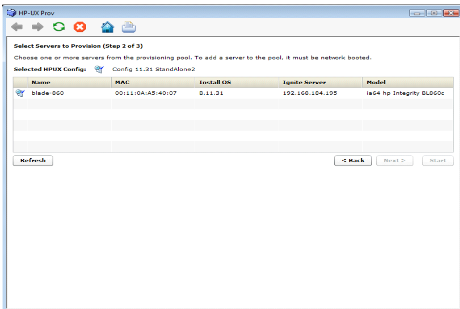
图 41.用于重新配置的已删除托管服务器列表
