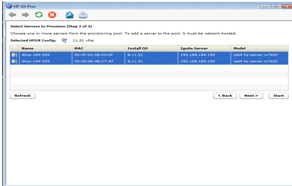
图 30.选择要使用之前的配置进行配置的客户端
