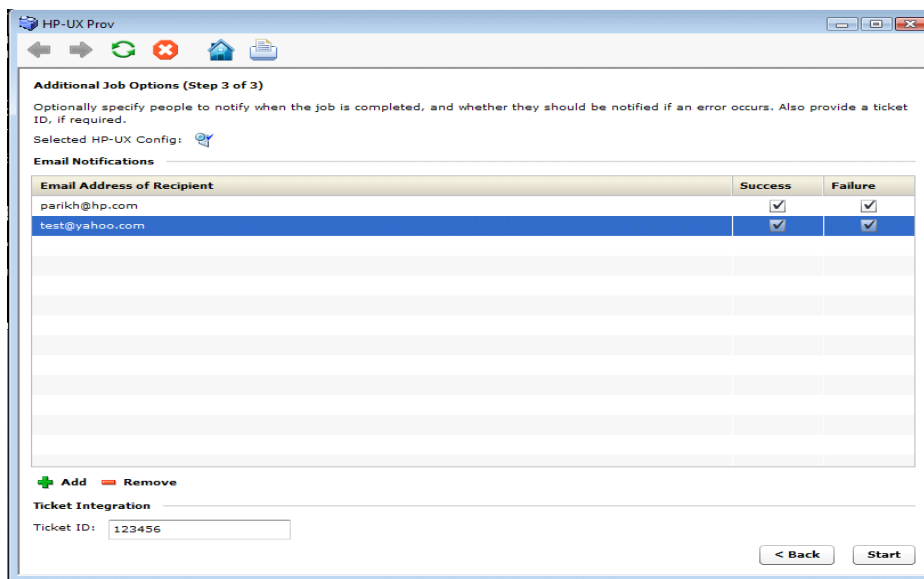
图 31.设置电子邮件通知
