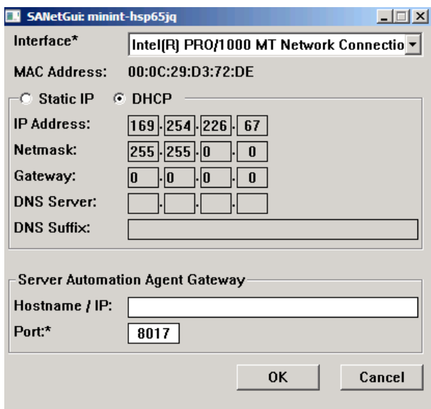
图 20.WinPE 网络配置
