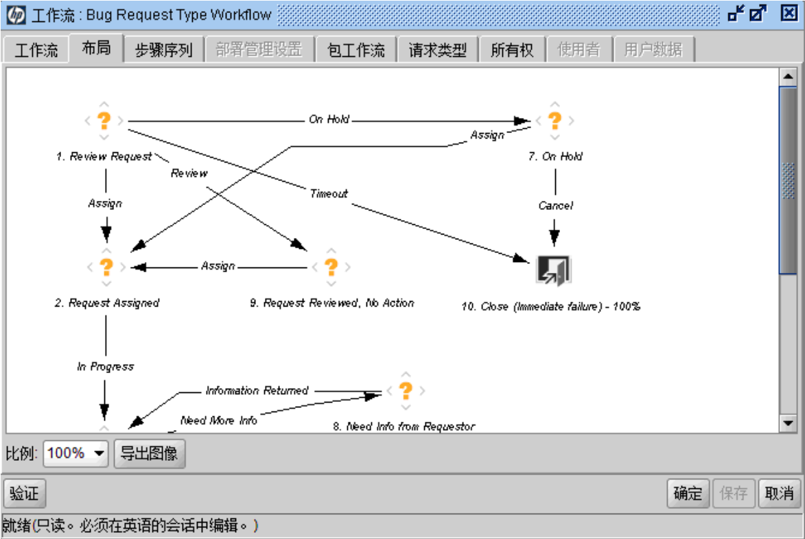
图 1-6. 包工作流
