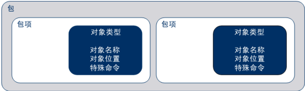
图 1-2. 包
