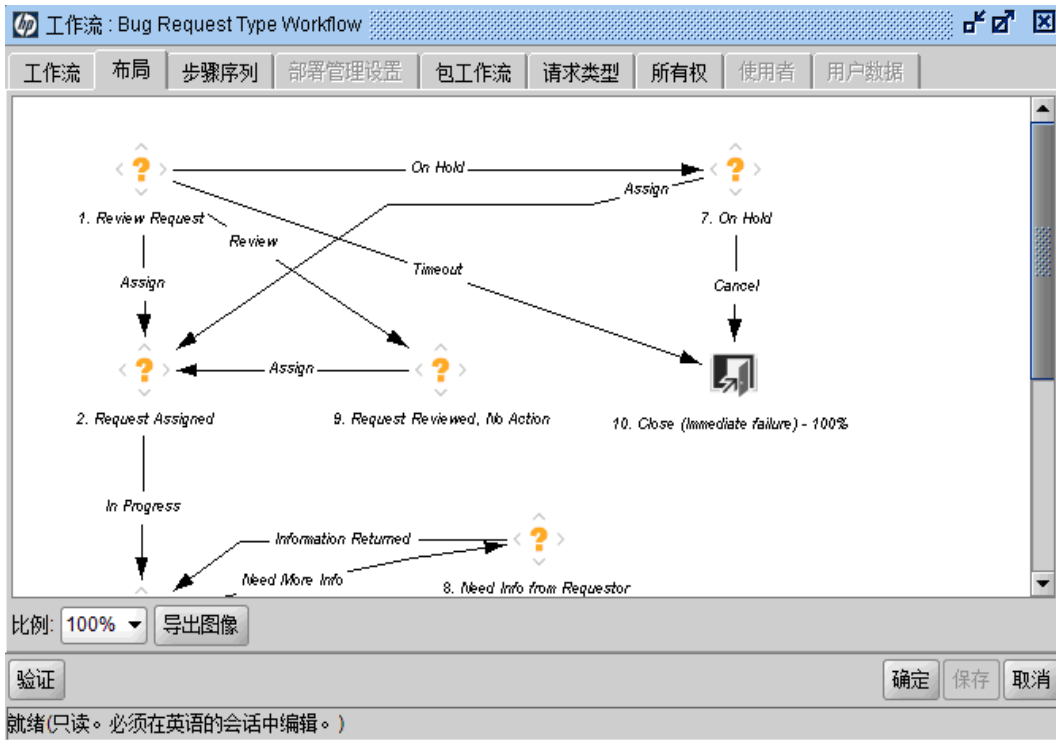
图 1-4. 包 workflow
