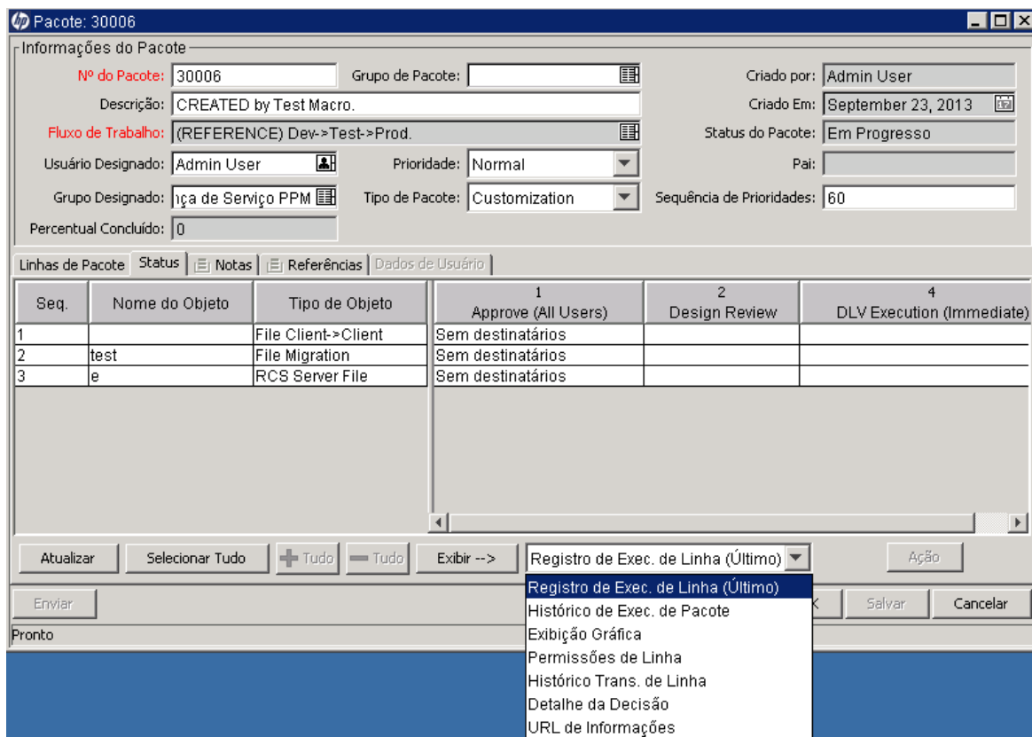
Figura 2-12. Janela Pacote, guia Status
