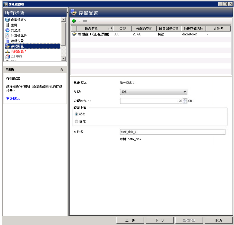
图 22 存储配置窗口 - SCVMM
