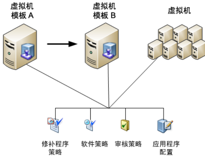
图 12 修改策略并创建新虚拟机模板
