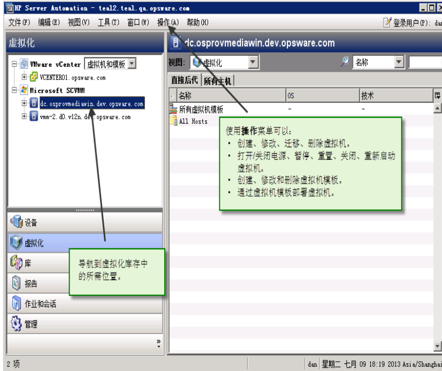
图 7 使用操作菜单管理 VS、虚拟机和虚拟机模板
