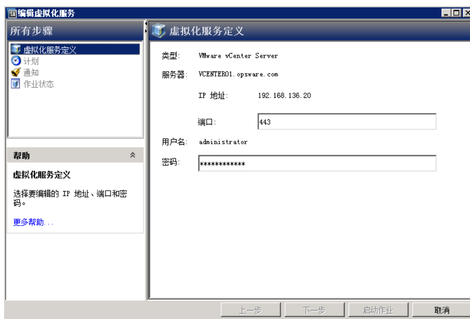
图 18 虚拟化服务定义窗口
