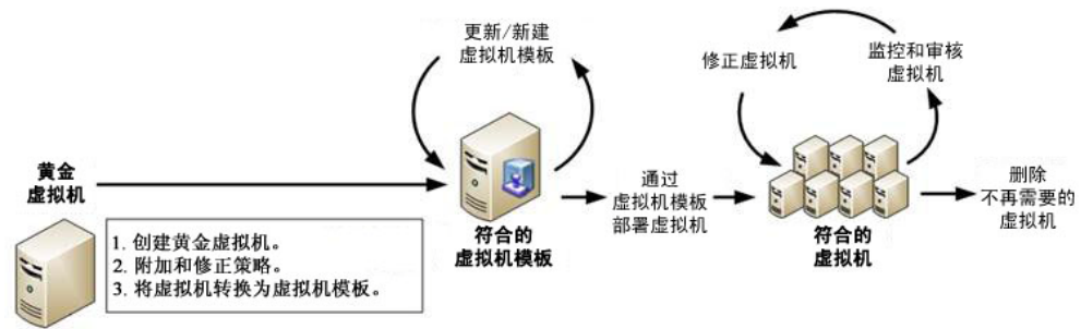
图 9 虚拟机生命周期
