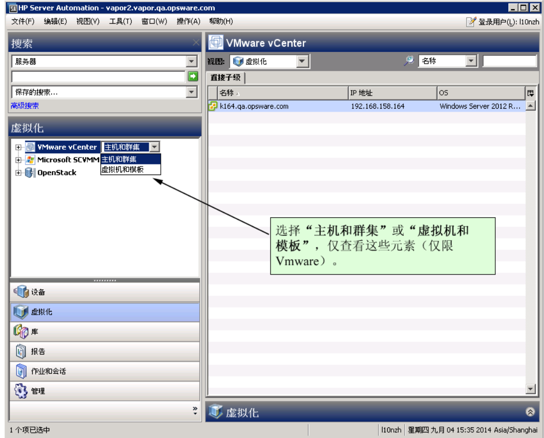
图 5 主机和群集视图、虚拟机和模板视图
