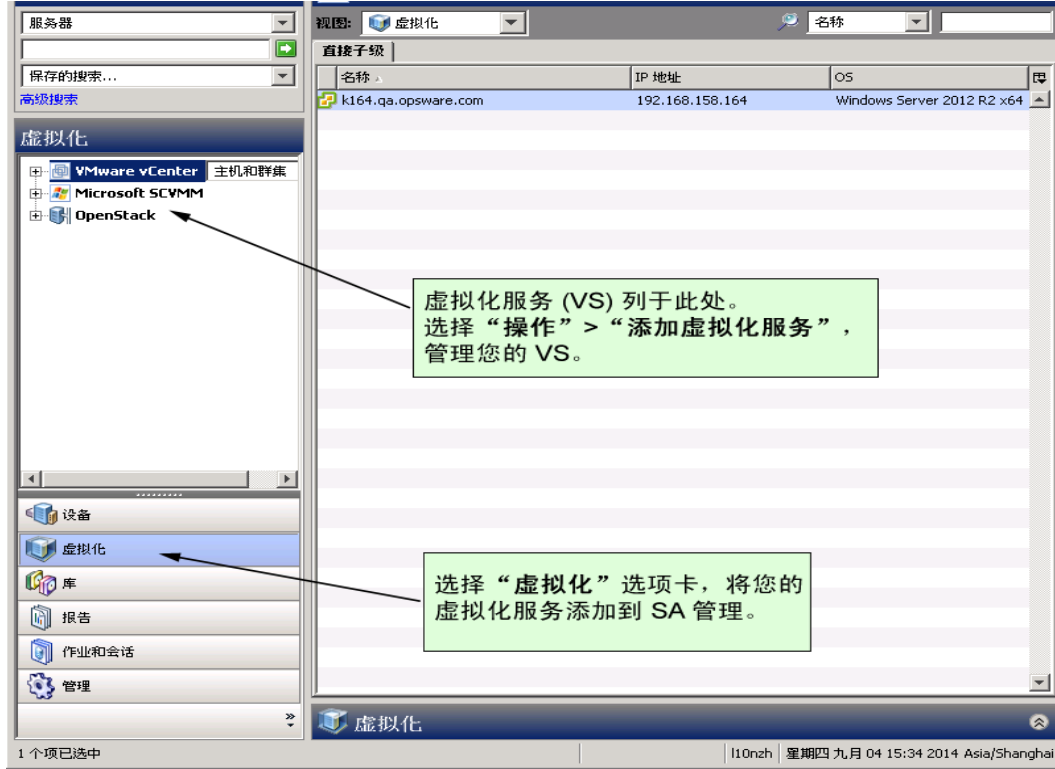
图 4 SA 客户端虚拟化选项卡
