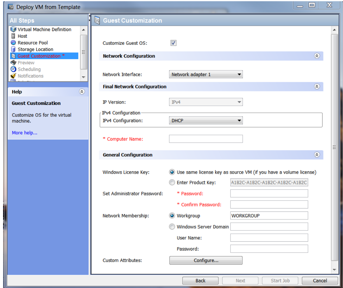
图 25 Windows 源的来宾自定义
