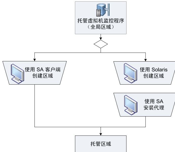
图 36 Oracle Solaris 区域上的 OS 配置和代理安装
