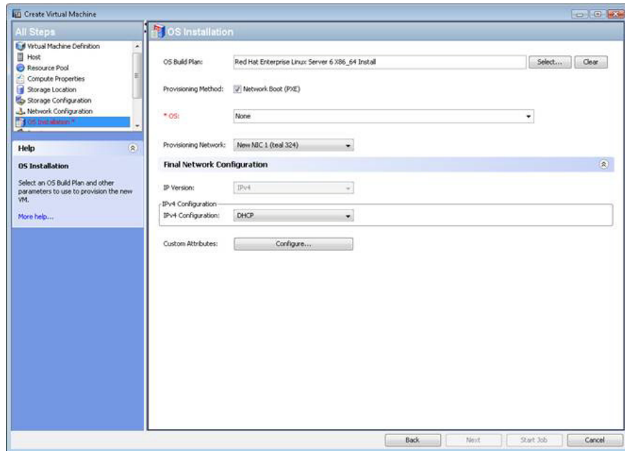
图 21 OS 安装窗口
