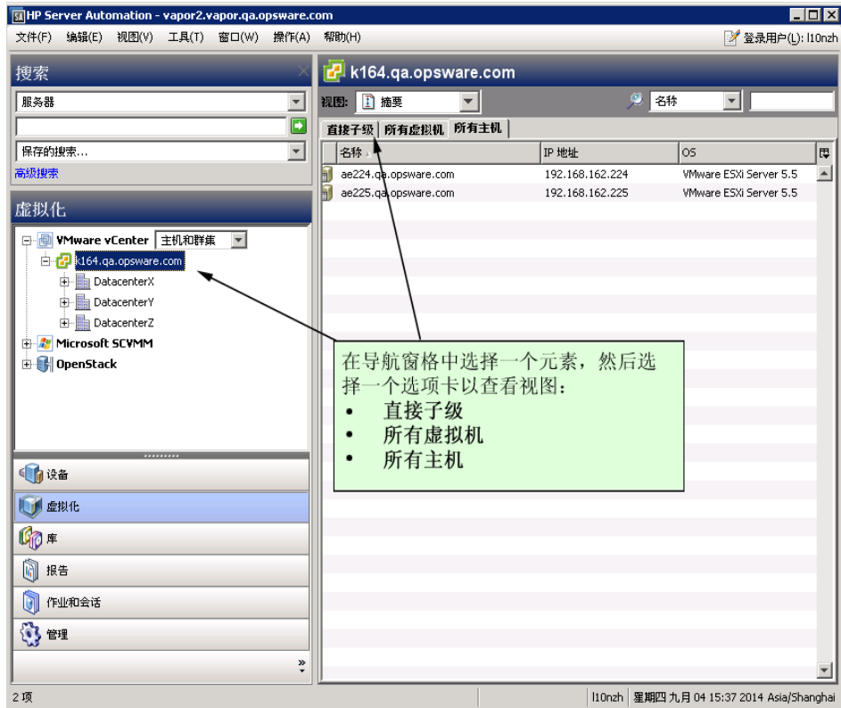
图 6 显示不同视图的选项卡
