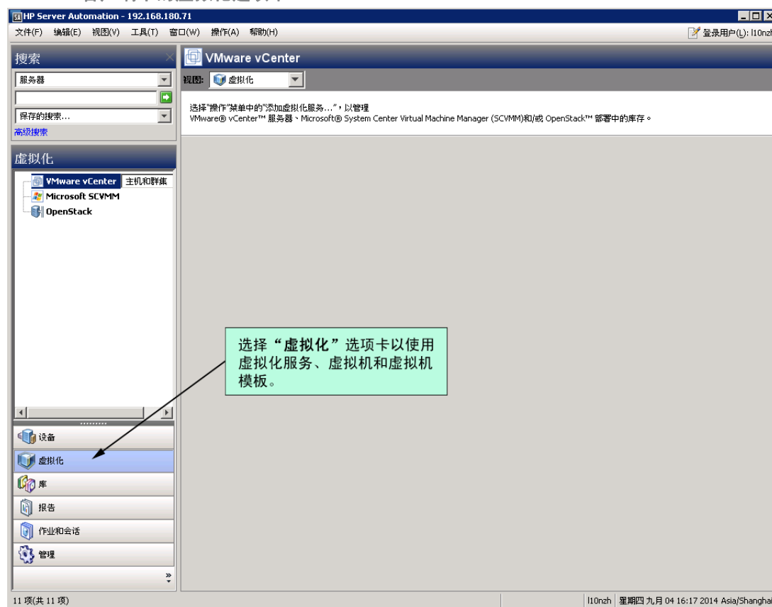
图 19 SA 客户端中的虚拟化选项卡
