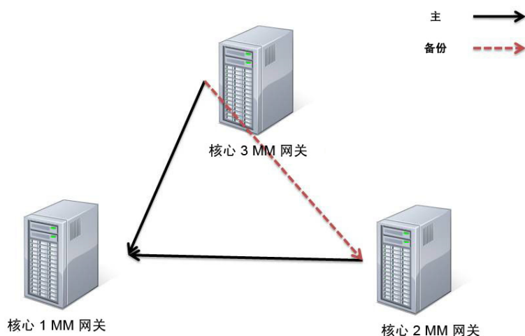
图 5 包含三个核心和一个备份路由的网状网络
