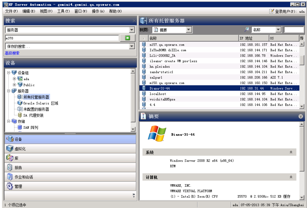
图 2 SA 客户端主屏幕
