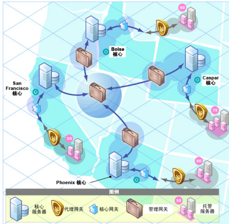
图 9 包含四个核心的多主控网状网络
