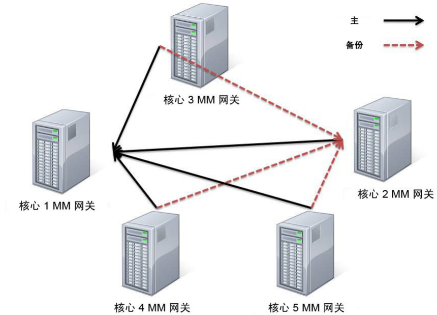
图 6 包含五个核心和多个备份路由的网状网络
