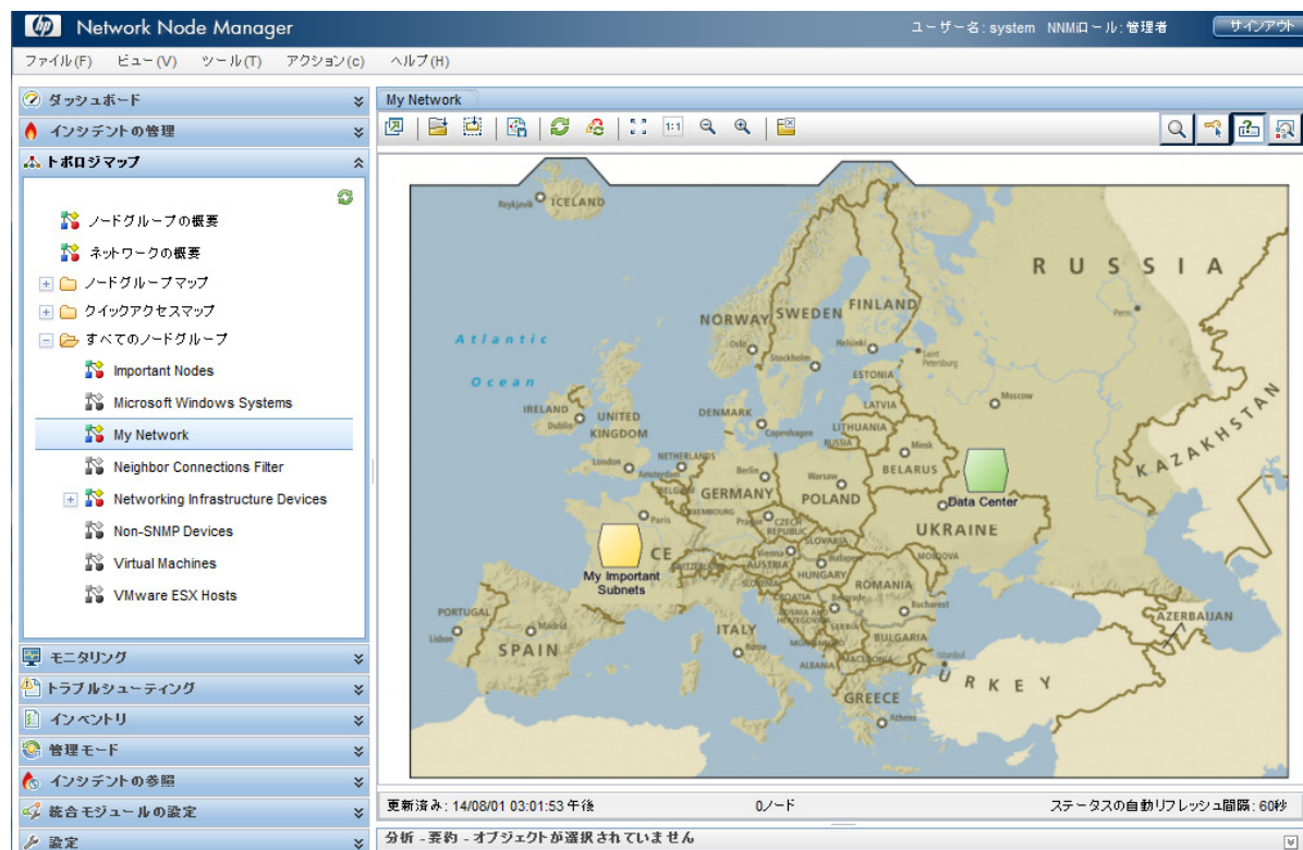
図 58: My Network マップ
