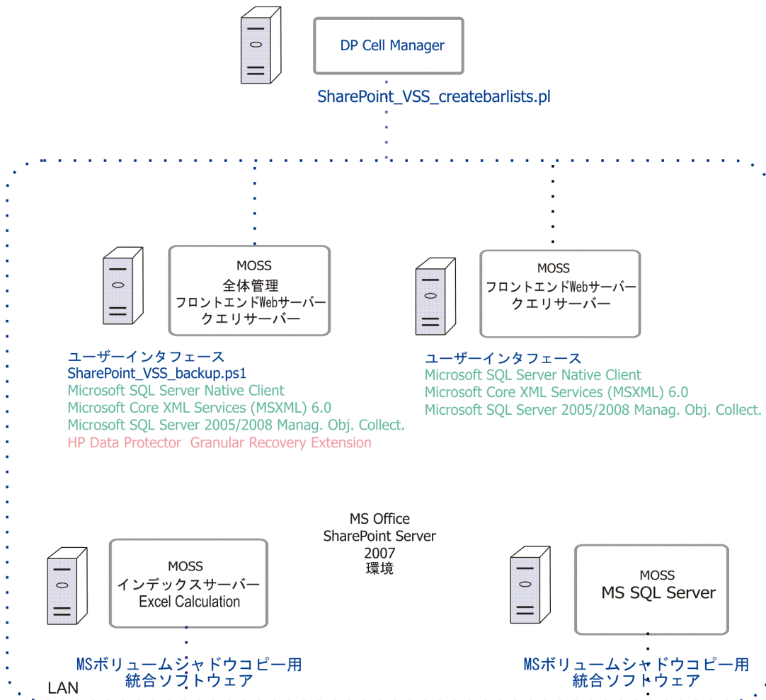
図 2 HP Data Protector Microsoft SharePoint Server VSS ベースソリューションを使用する中規模ファームのインストール (例)
