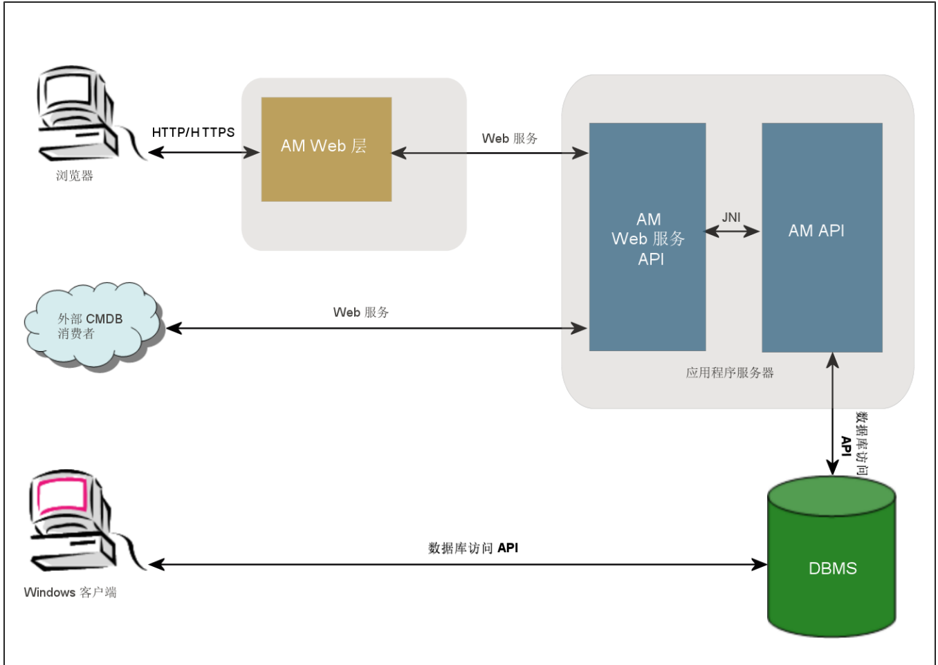
Asset Manager Web 体系结构
