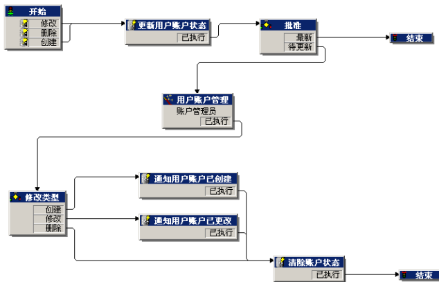
用户账户管理工作流 - 关系图
