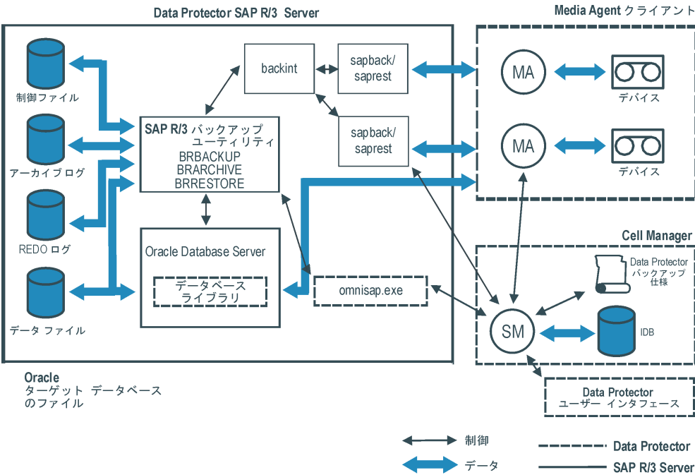
図 29 SAP R/3 のアーキテクチャ
