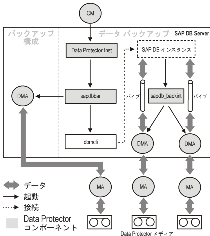
図 43 SAP DB 用統合ソフトウェアのアーキテクチャ
