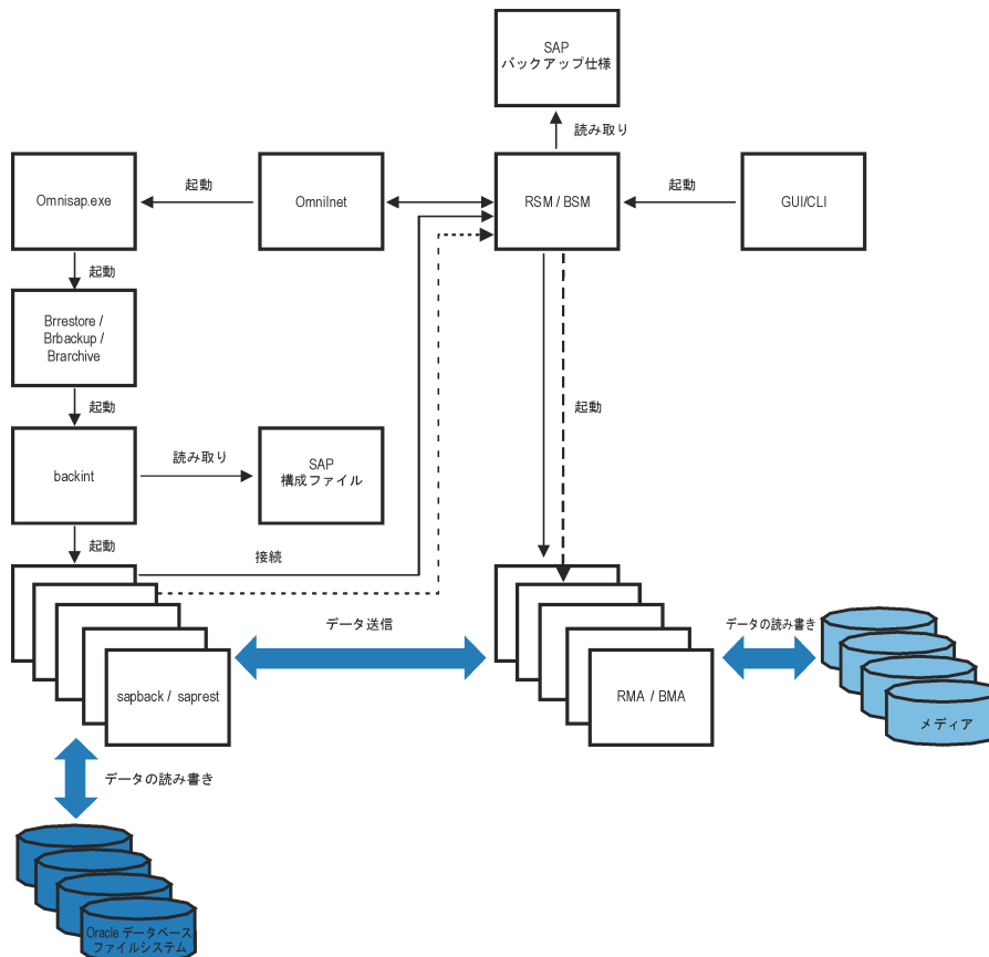
図 30 SAP R/3 のアーキテクチャ:backint モード
