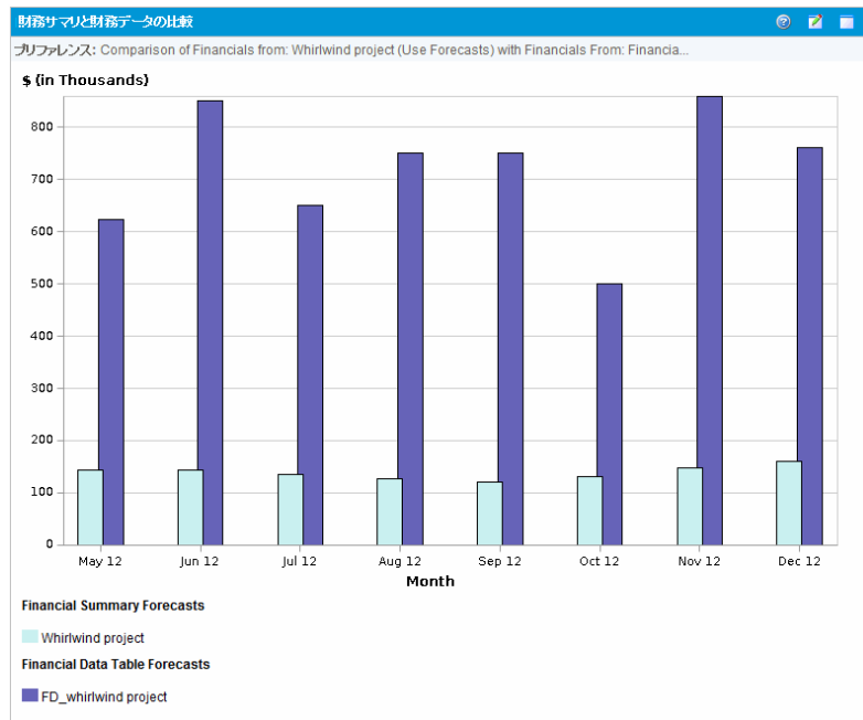
図 4-14. 予測の比較
