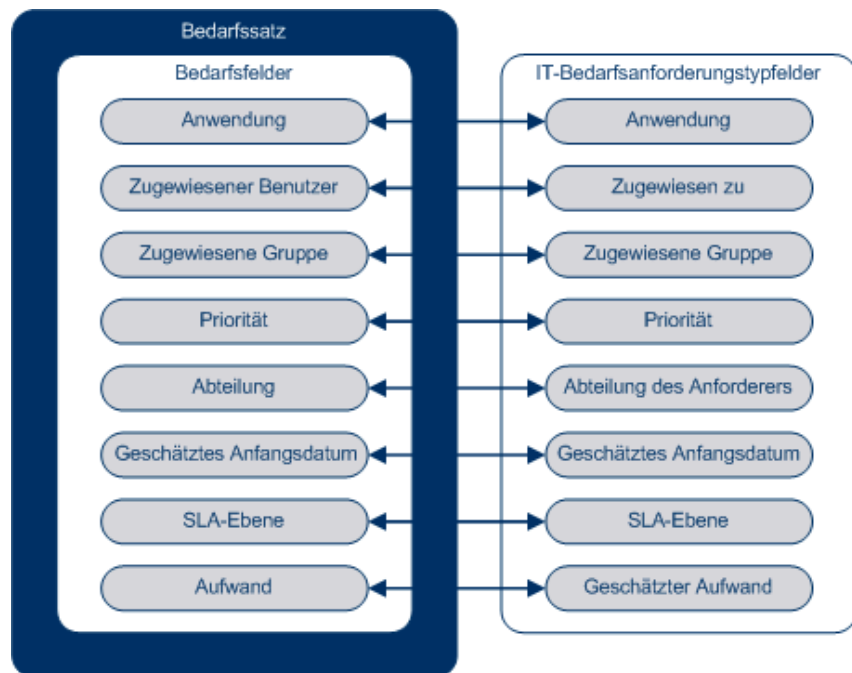
Abbildung 1-2. Zuordnung von Bedarfssatz- und IT-Bedarfsanforderungstypfeldern
