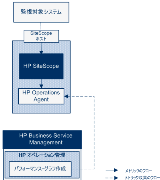
HP Operations Agent を使用した オペレーション管理へのメトリクス・データ・フロー
