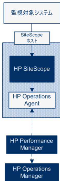
HP Operations Agent を使用した HPOM へのメトリクス・データ・フロー
