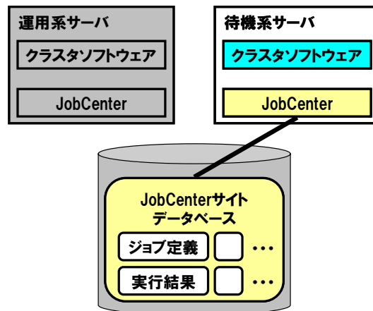
図 2-5 クラスタ環境でのサイト動作図 4
