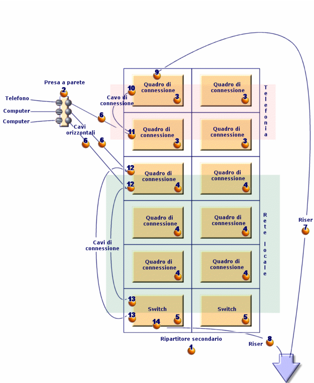
Figura 2.2. Esempio pratico - rete cablata da rappresentare
