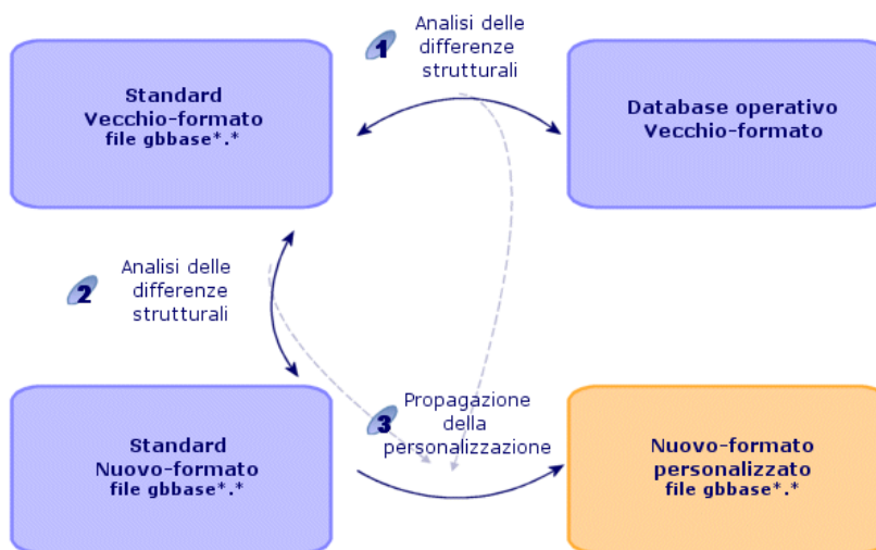
Figura 4.1. Diffusione dei cambiamenti strutturali - procedimento
