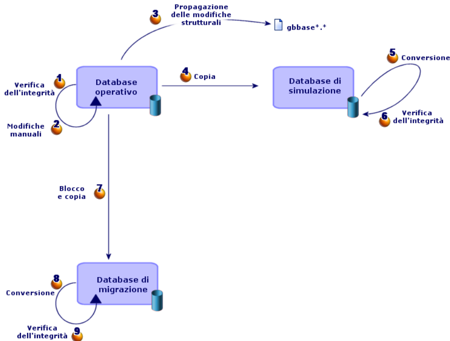
Figura 2.2. Conversione - procedura per convertire AssetCenter versione 4.2.x
