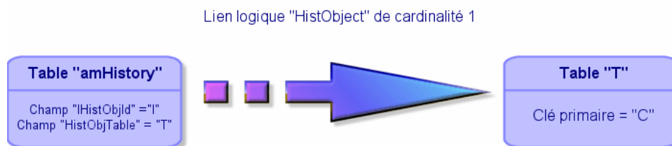
Figure 2.3. Liens entre la table des historiques et une table cible
