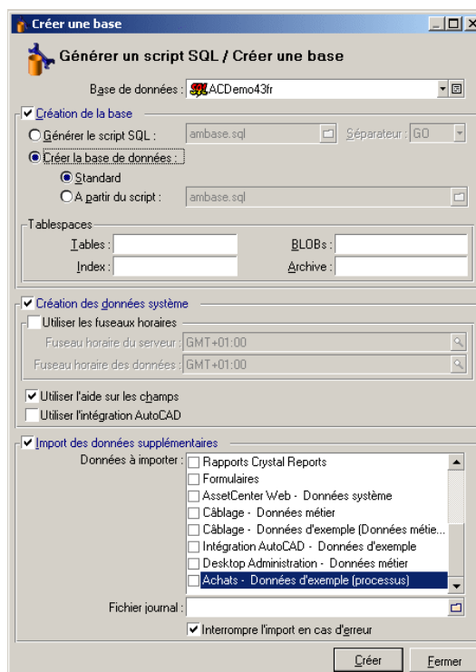
Figure 3.1. Base de données - fenêtre de création
