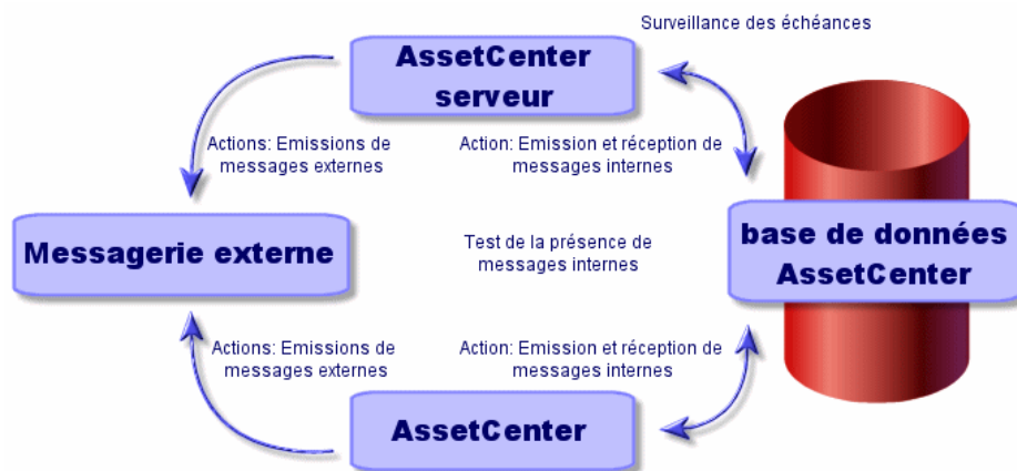
Figure 14.1. Messagerie - fonctionnement général
