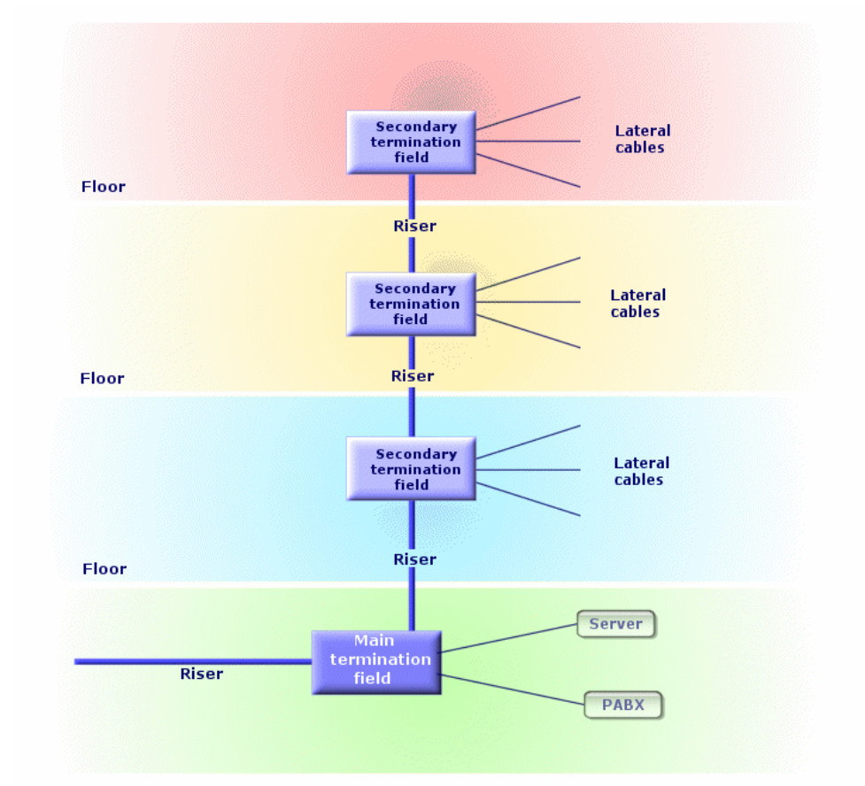
Abbildung 8.9. Vertikale Verteilung eines verkabelten Netzes - Darstellung
