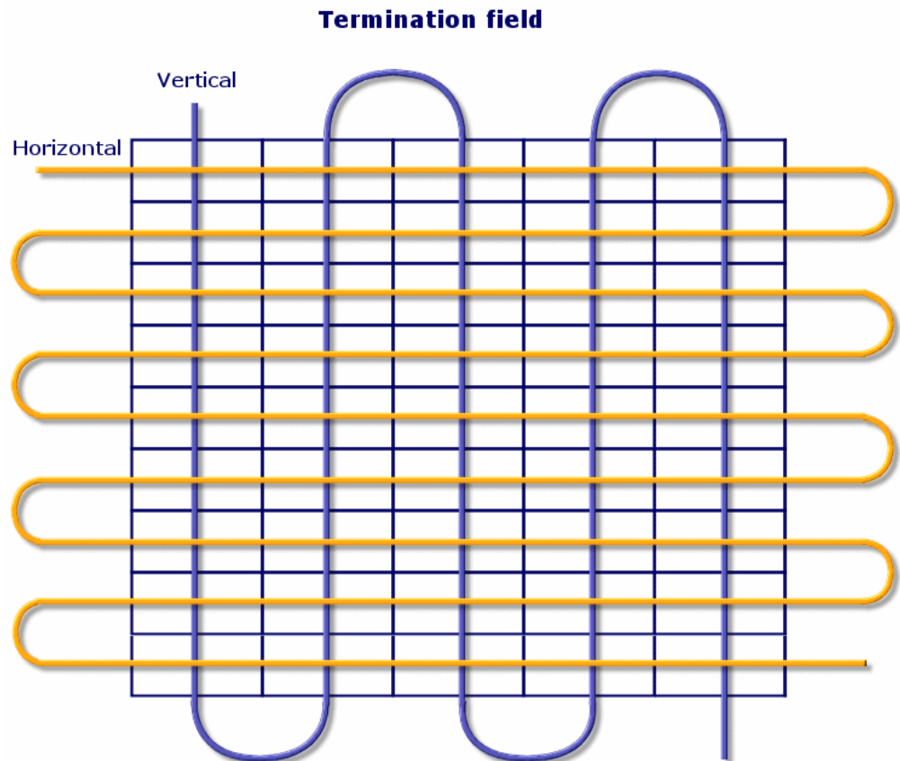
Abbildung 3.19. Verteilerkonfiguration - Bedeutung der Bestückungsrichtung
