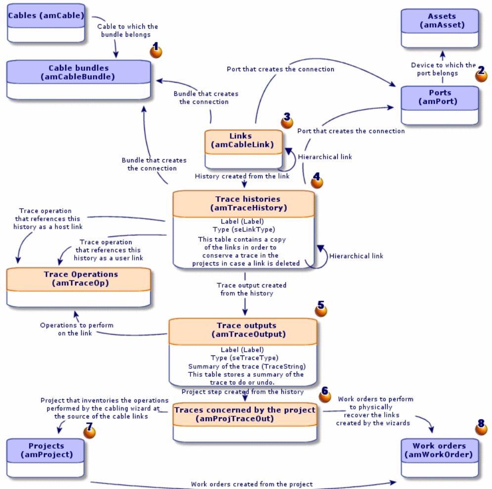
Abbildung 5.9. Verbindungen - detailliertes Datenmodelle
