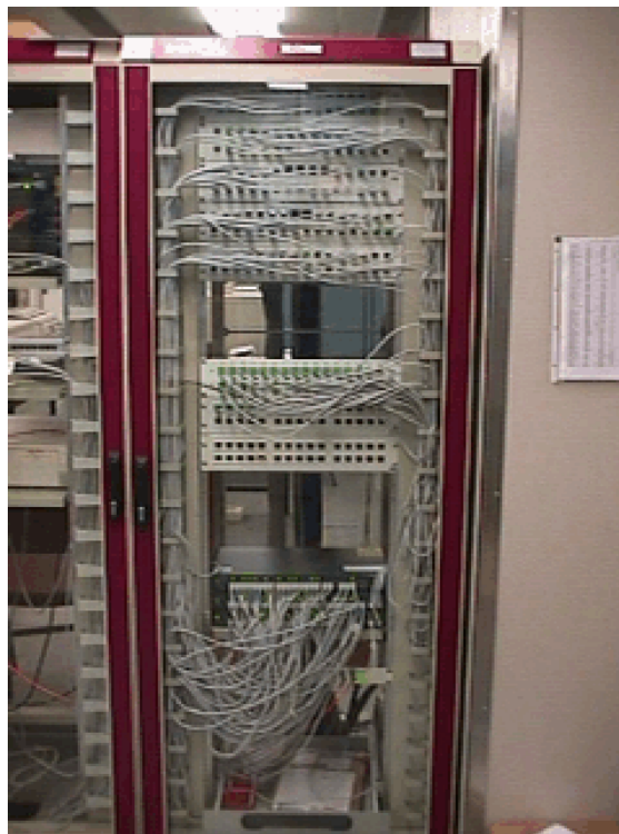
Abbildung 8.7. Steckschrank - Foto
