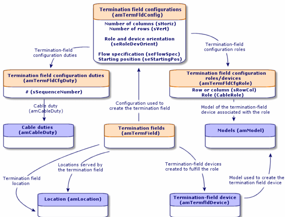
Abbildung 3.12. Verteilerkonfigurationen - Datenmodell
