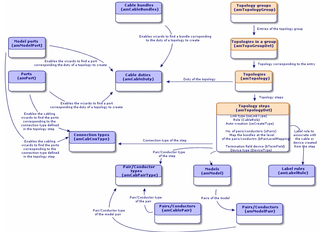
Abbildung 3.9. Topologien - Datenmodell
