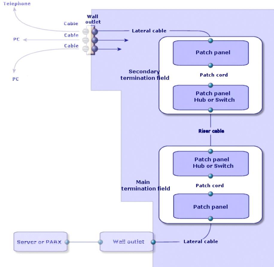
Abbildung 1.1. Vom Modul Kabel abgedeckter Bereich
