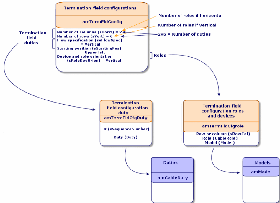
Abbildung 3.13. Beispiel für eine Verteilerkonfiguration - Darstellung in der AssetCenter-Datenbank.
