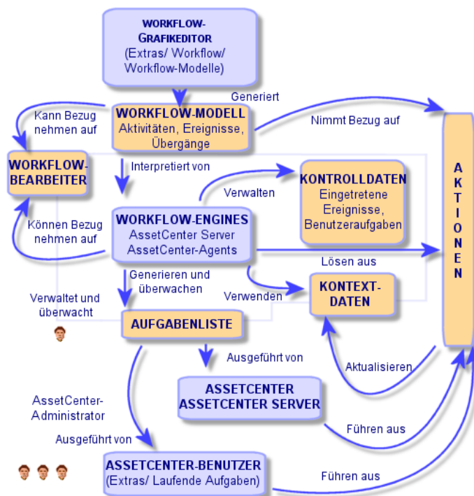
Abbildung 8.2. AssetCenter-Workflow - Allgemeine Übersicht
