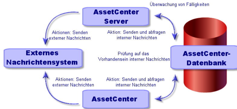
Abbildung 7.1. Nachrichtensystem - Allgemeine Funktionsweise
