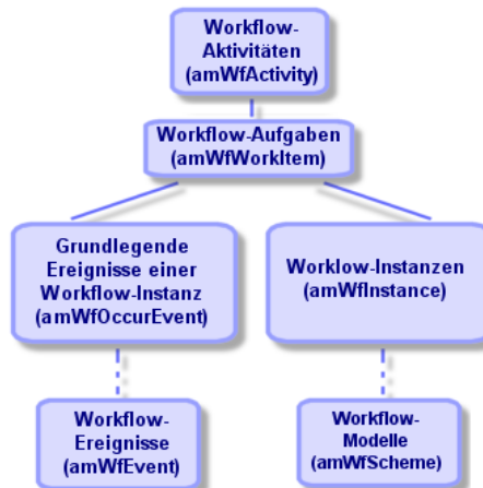
Abbildung 8.4. Workflow - Im Rahmen des Ablaufs einer Workflow-Instanz hauptsächlich verwendete Tabellen
