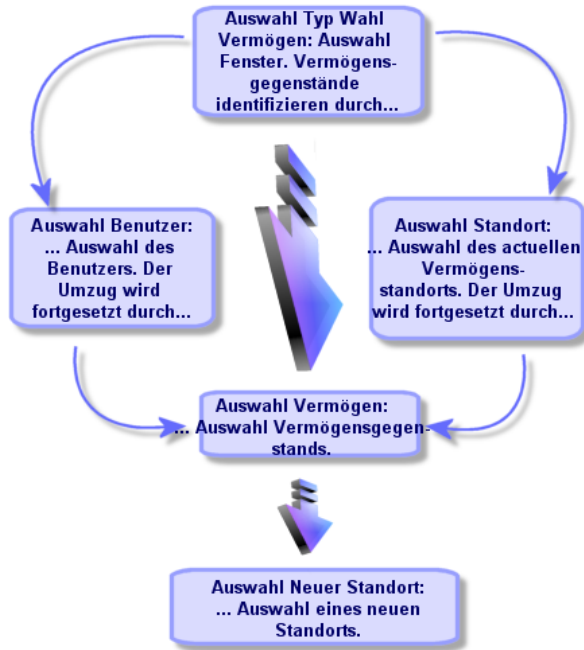
Abbildung 14.3. Assistent - Beispiel
