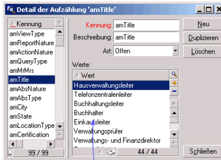
Abbildung 1.1. Aufzählung - Fenster
