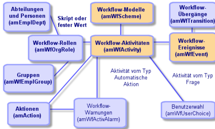
Abbildung 8.3. Workflow - Zum Definieren eines Workflow-Modells hauptsächlich verwendete Tabellen
