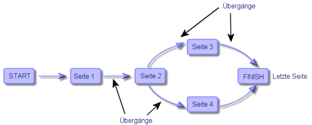
Abbildung 14.1. Assistenten - Strukturmodell
