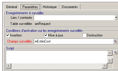
Figure 8.7. Onglet Paramètres d'un événement de type Base
