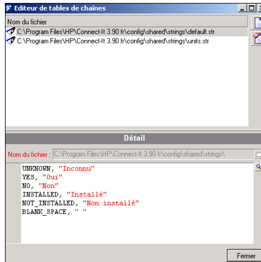
Figure 4.17. L'éditeur des tables de correspondance
