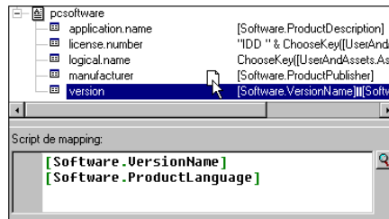
Figure 4.19. Glisser-déplacer plusieurs champs
