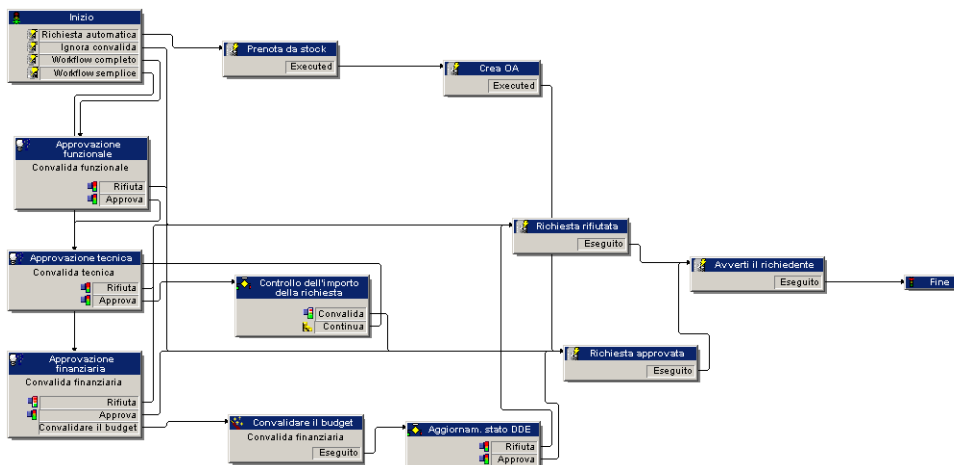
Figura 6.2. Schema di workflow della convalida della richiesta di acquisto
