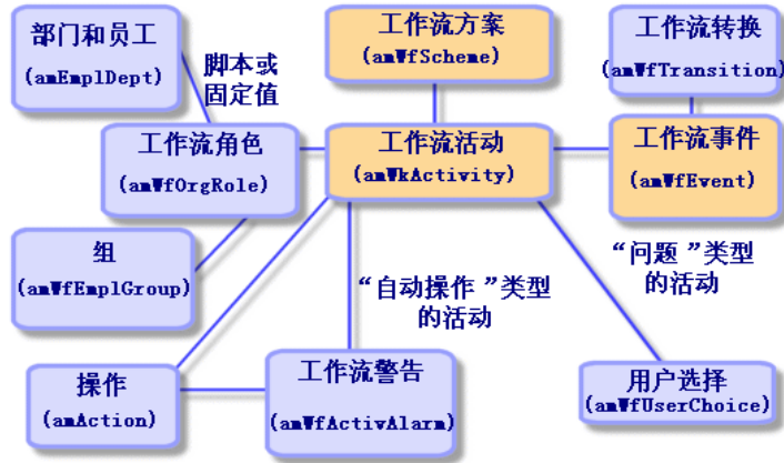
图 8.9. 工作流 - 定义工作流方案的主表
