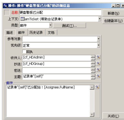
图 7.3. 链接到升级方案的邮件输入操作 - 详细信息窗口
