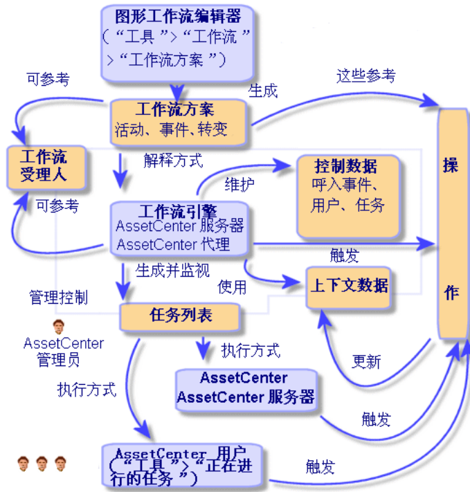
图 8.2. Asset Manager 中的 workflow - 概述
