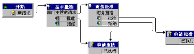
图 8.4. workflow - 申请审批方案
