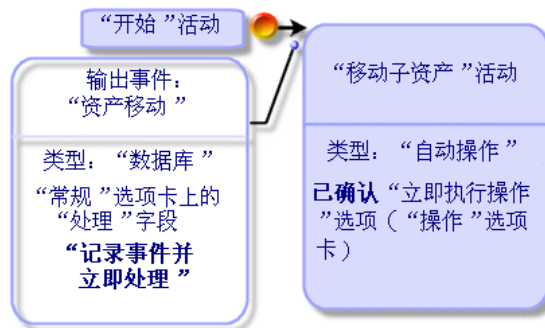
图 8.6. 同步 workflow 方案示例
