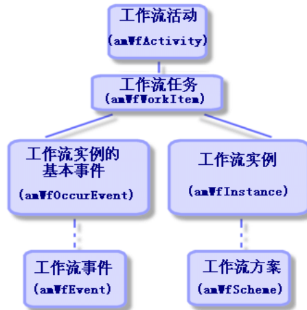
图 8.10. 工作流 - 执行中的工作流实例所涉及的主表
