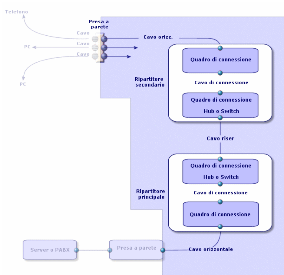
Figura 1.1. Modulo Cablaggio - aree gestite
