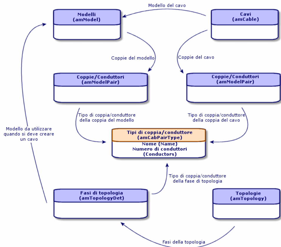
Figura 3.4. Tipo di coppia/connettore - modello dati
