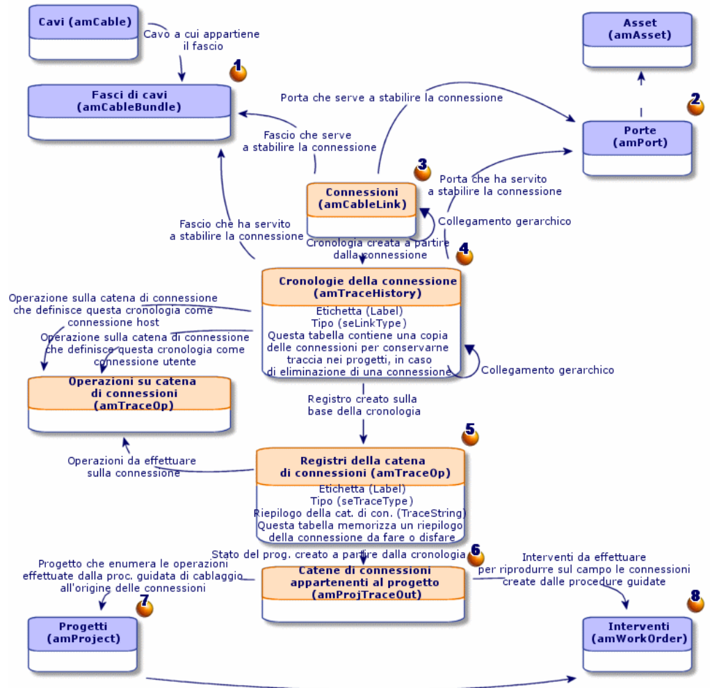
Figura 5.9. Connessioni - modello dati dettagliato
