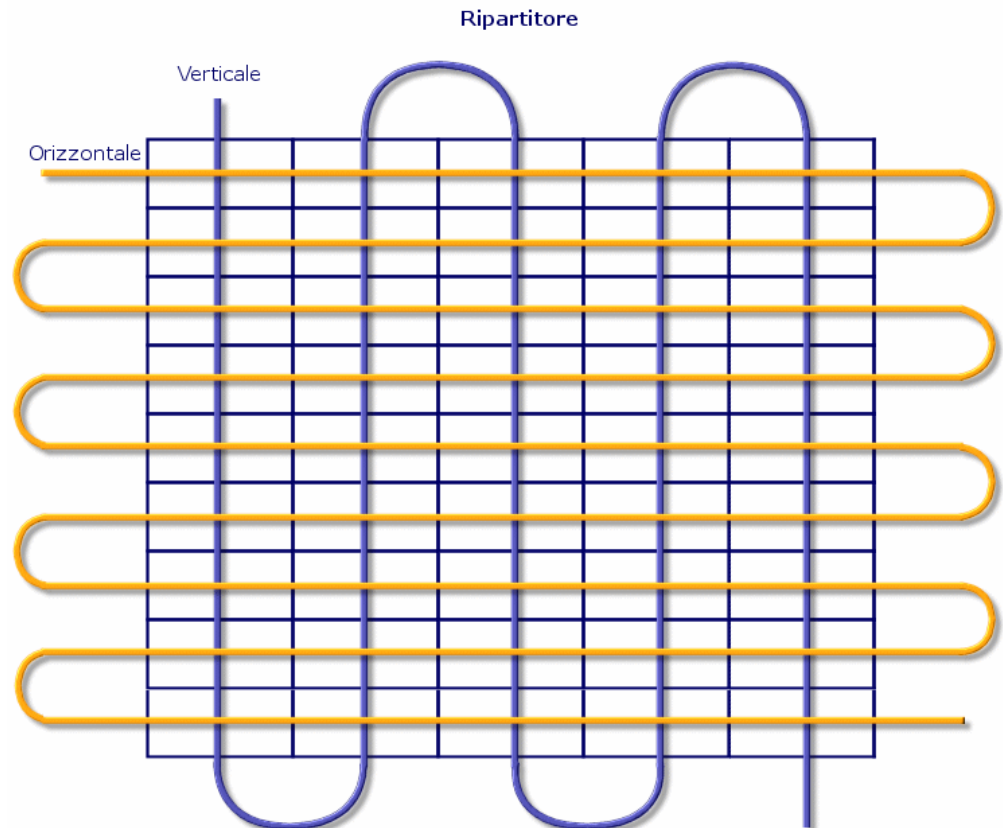
Figura 3.19. Configurazione ripartitore - significato del senso di completamento
