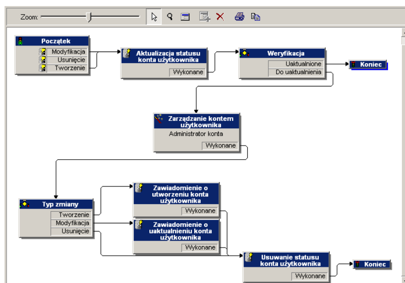
Rysunek 7.1. Workflow Zarządzanie kontem użytkownika - schemat
