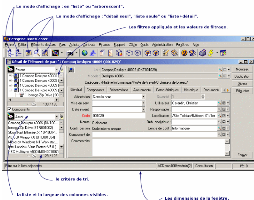
Figure 5.1. Les éléments mémorisés d'une vue
