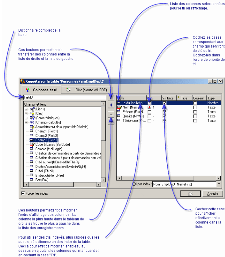
Figure 2.4. Configuration d'une liste
