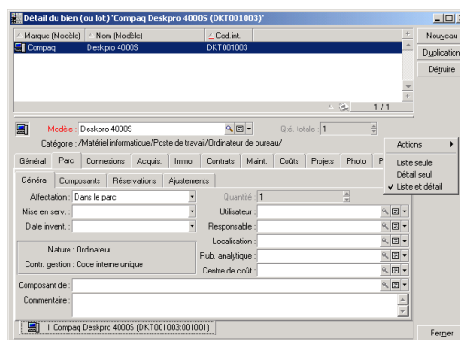
Figure 2.6. Affichage combiné de la liste des biens et d'un détail
